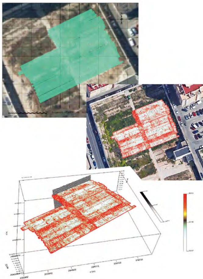
Fig. 47 | Prospección con georradar multicanal 3D en las fosas del Patio 1.º (U.A.U.C.M.).
