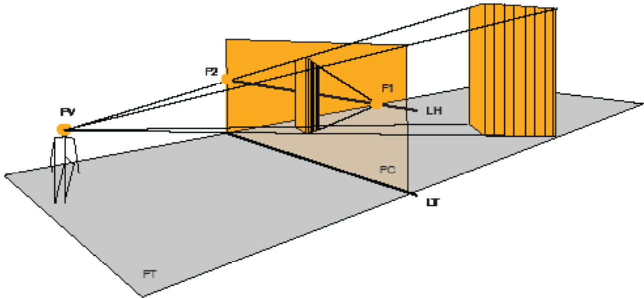
Fig. 3.5: Elementos de la perspectiva Fuente: Salinas (2017)
