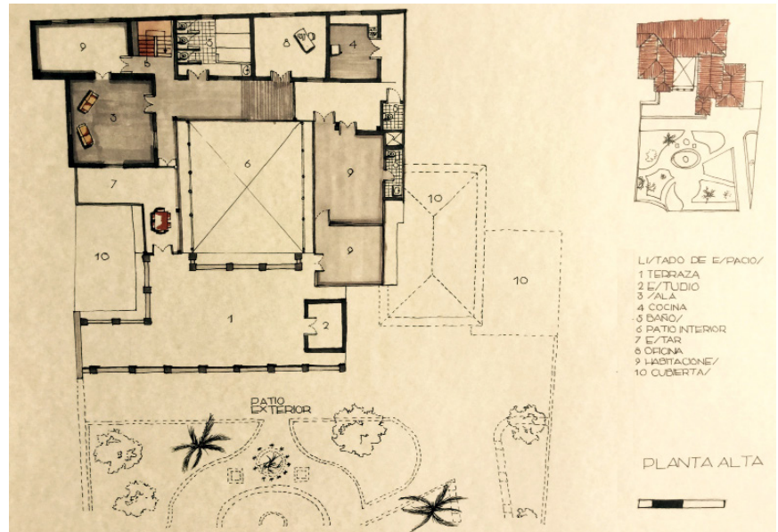
Fig. 4.6: Planta alta de la Quinta Guadalupe
