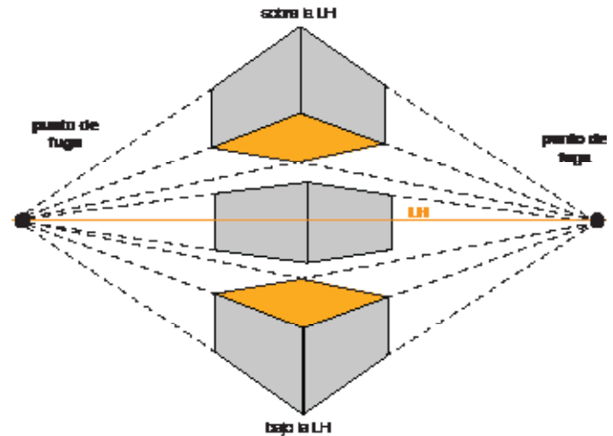
Fig. 3.14: Esquema de la perspectiva con dos puntos de fuga Fuente: Salinas (2017)
