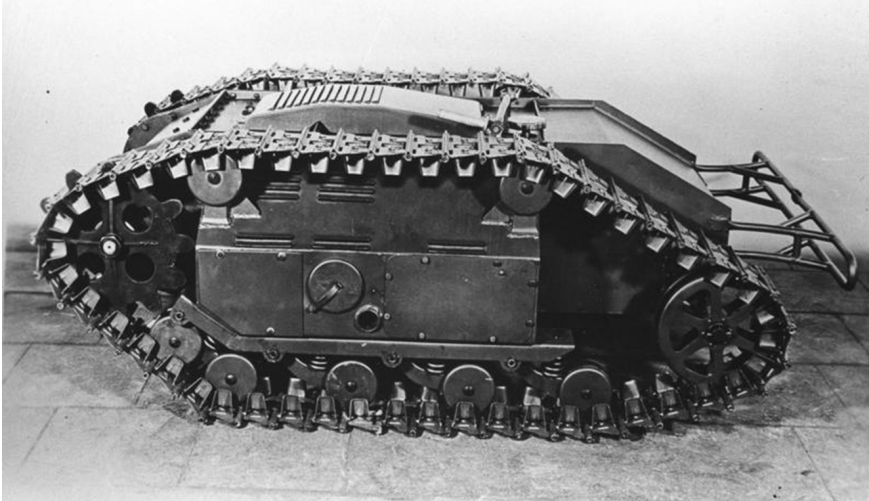
Figura 1.4. Vehículo teledirigido Goliath. Fotografía realizada en hacia 1943-1944 (fuente: Deutsches Bundesarchiv, https://goo.gl/ZoYUgx ).
