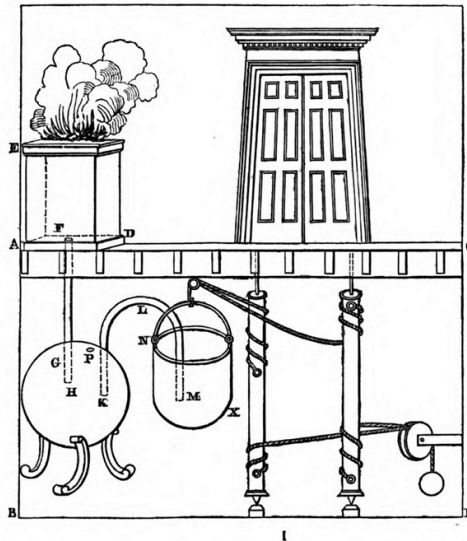
Figura 1.1. Mecanismo para la apertura automática de puertas (Herón de Alejandría. Pneumatika . Traducción de Bennet Woodcroft, Londres: Taylor Walton and Maberly, 1851).
