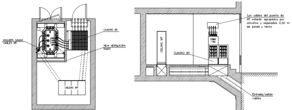
Solución CT fachada estrecha
