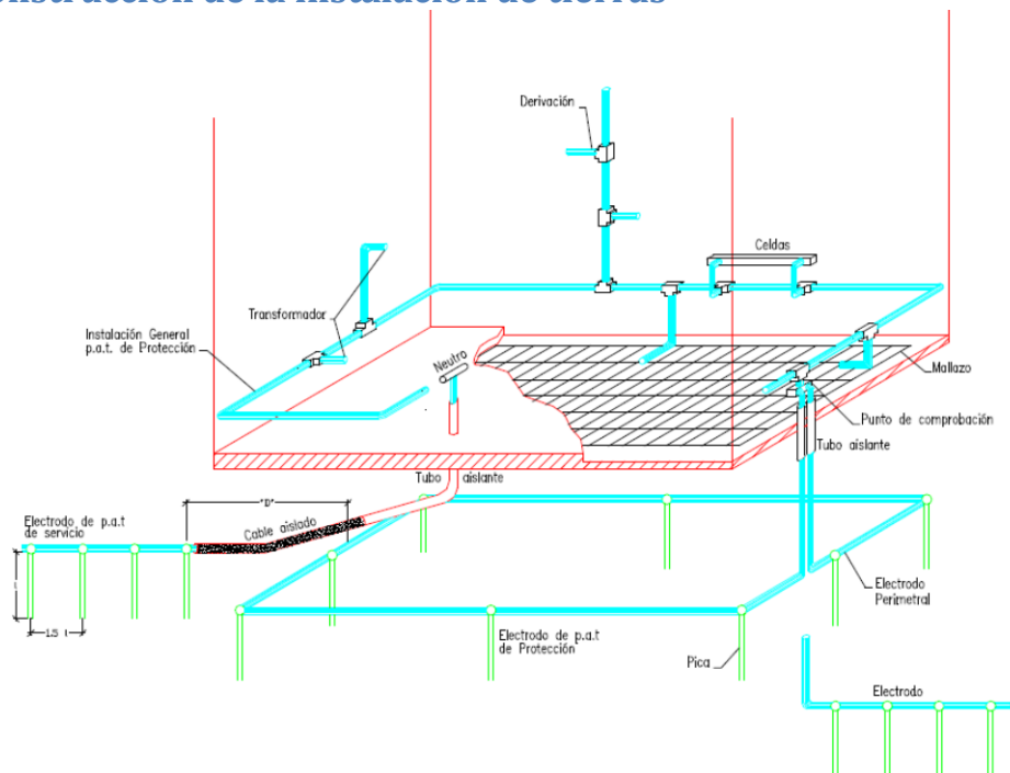
Instalación de puesta a tierra
