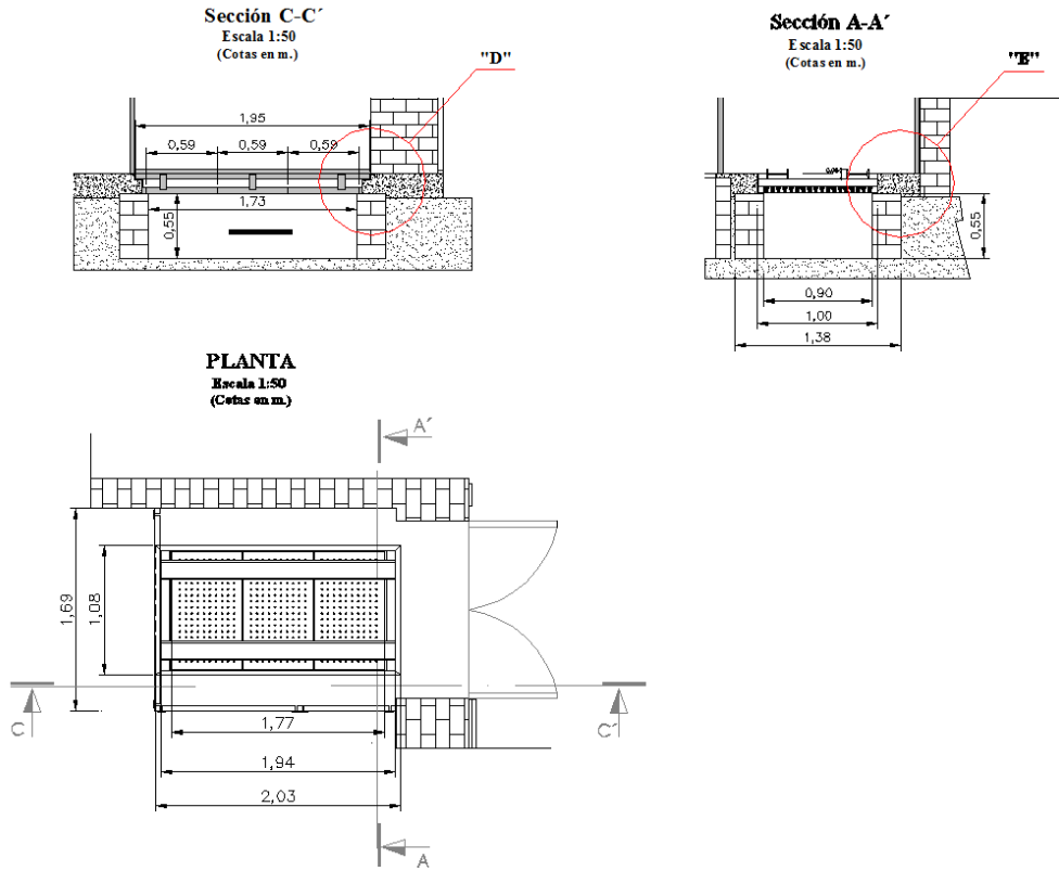
FIGURA: Detalle de foso
