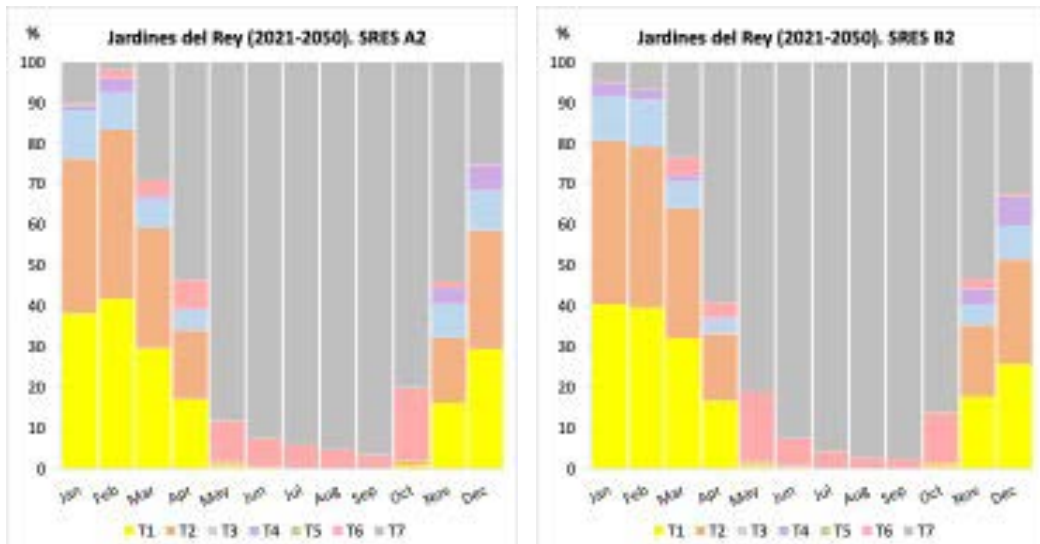
Figura N° 2 Distribución anual de los tipos de tiempo en Jardines del Rey (2021-2050 base diaria, escenarios A2 y B2).
