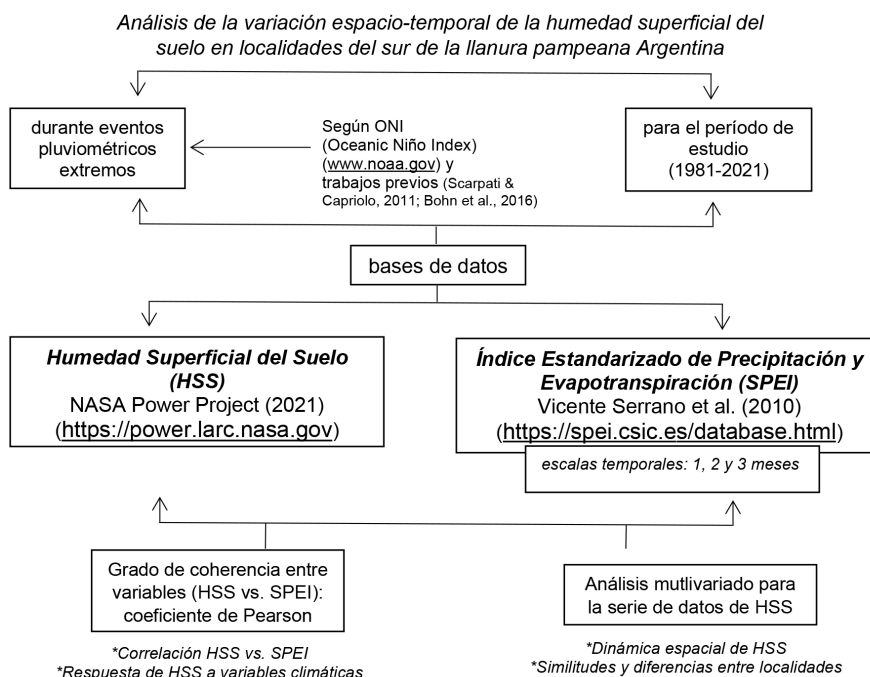
Figura 2. Diagrama metodológico
