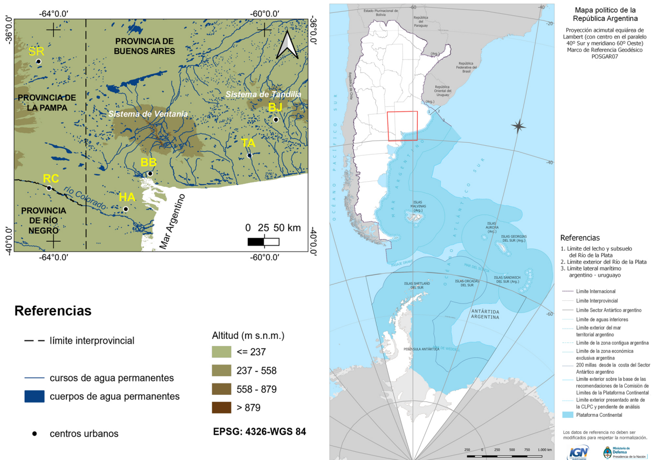
Figura 1. Localidades analizadas y aspectos físico-geográficos de la región de estudio: BJ, Benito Juárez; TA, Tres Arroyos; BB, Bahía Blanca; HA, Hilario Ascasubi; RC, Río Colorado; SR, Santa Rosa
