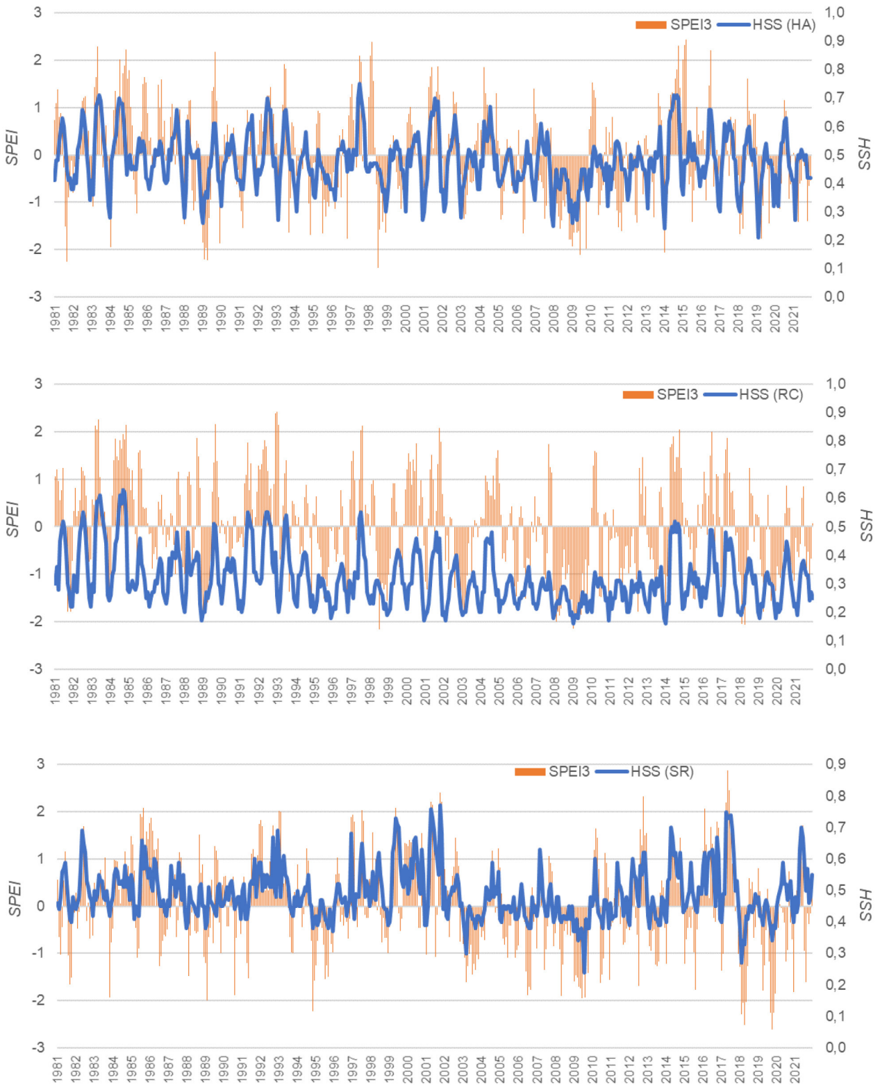
Figura 4. Evolución temporal interanual de la HSS durante el período estudiado (1981-2021) e índice climático SPEI a escala 3 meses, para cada localidad (de este a oeste): HA, Hilario Ascasubi; RC, Río Colorado SR, Santa Rosa
