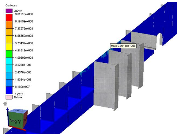
Figura 16. Tensiones máximas de von Mises (Pa) en la cubierta principal del modelo del MEF para el caso de carga II con la pluma de la grúa en una posición de 90°.
