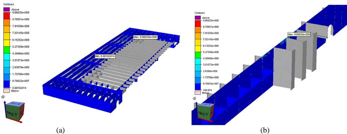
Figura 15. Tensiones máximas de von Mises (Pa) en la cubierta principal del modelo del MEF para el caso de carga I con la pluma de la grúa en una posición de 90°.
