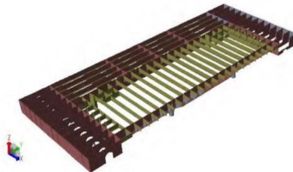
Figura 5. Modelo del MEF de la estructura interna de la cubierta principal de un buque de apoyo a plataformas.
