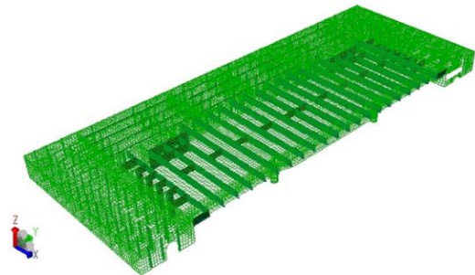
Figura 13. Mallado del modelo del MEF de la estructura interna de la cubierta principal del buque de apoyo a plataformas.
