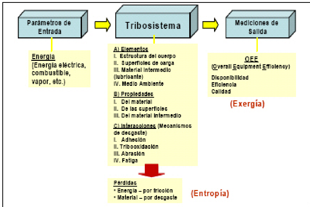
Fig. 5. Análisis tribotermodinámico de un tribosistema
