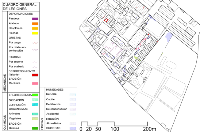
Figura 9: Estado patológico del inmueble Barbones (Cuartel de Caballería) y alrededores.
