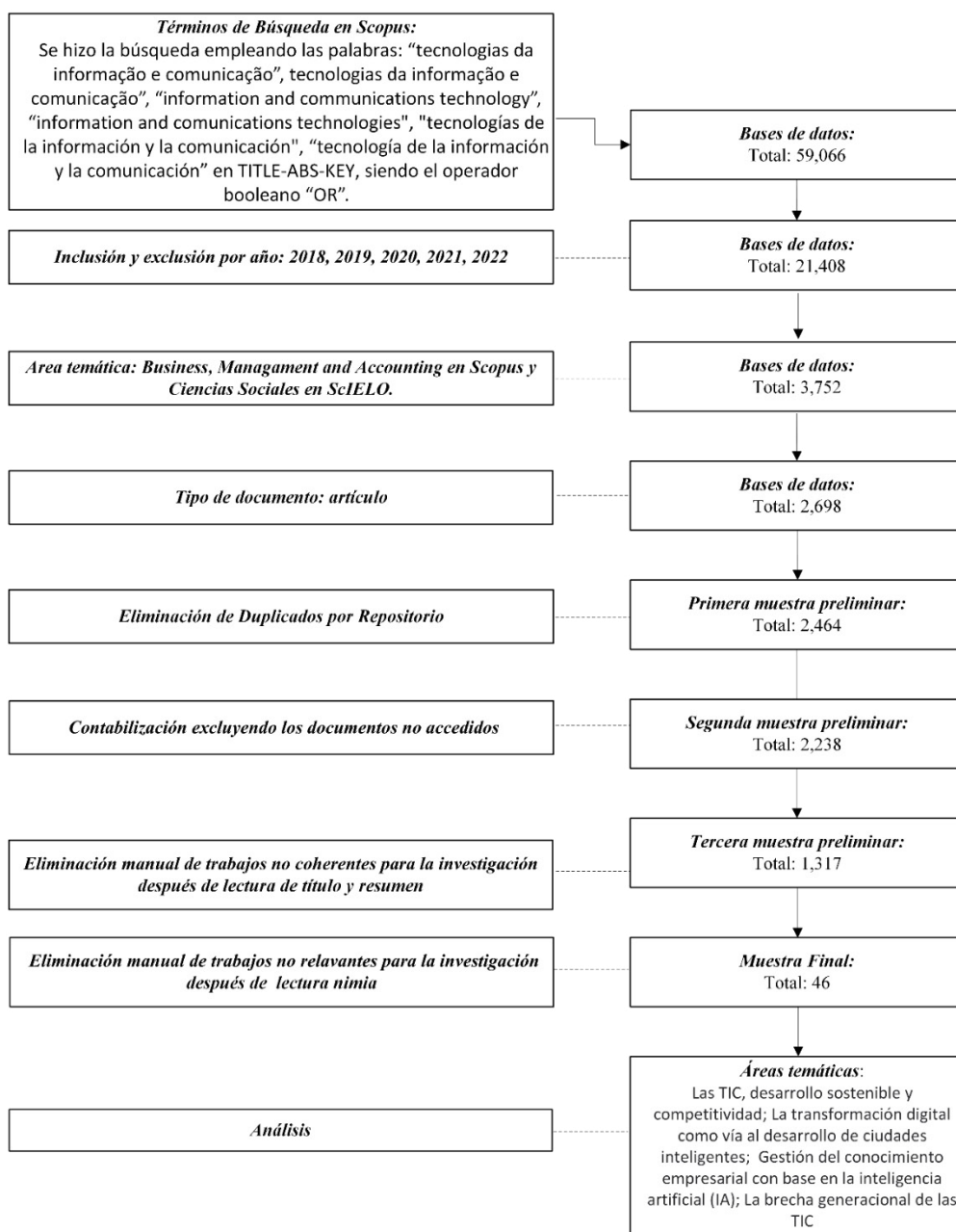
Figura 1. Método PRISMA
