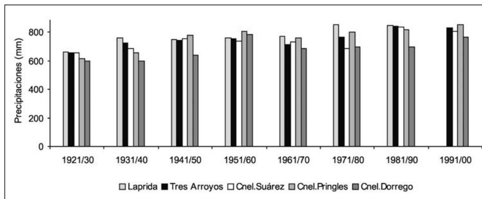
FIGURA 4 Evolución de las precipitaciones en ocho décadas y en cinco localidades de la cuenca
