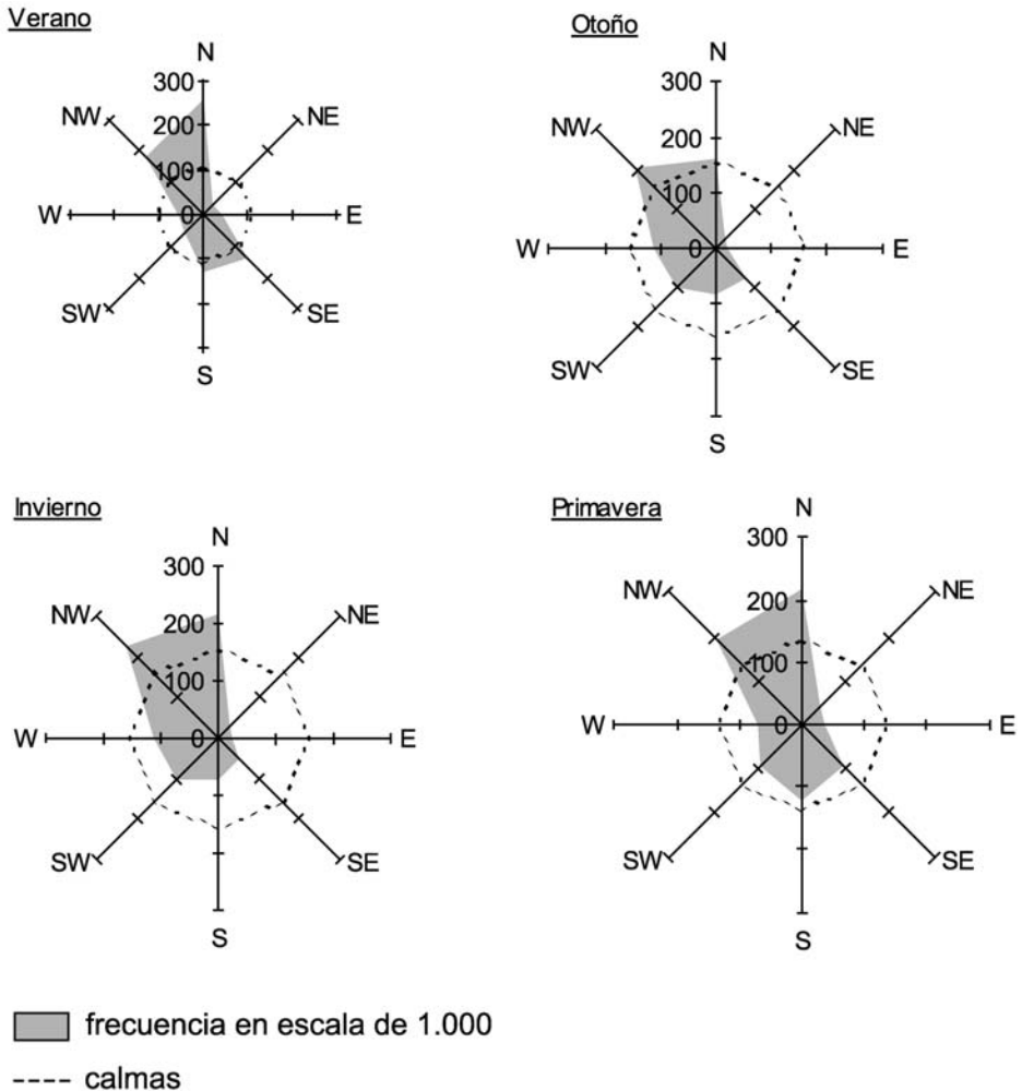
FIGURA 15 Rosas de vientos estacionales para Tres Arroyos. Período 1981/1990
