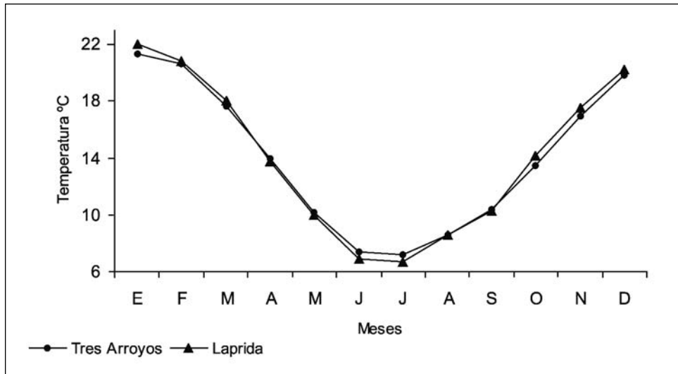
FIGURA 8 Temperatura media mensual de Tres Arroyos y Laprida 1981/1990
