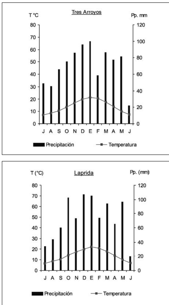
FIGURA 10 Diagramas Ombrotérmicos de Tres Arroyos y Laprida 1981/1990
