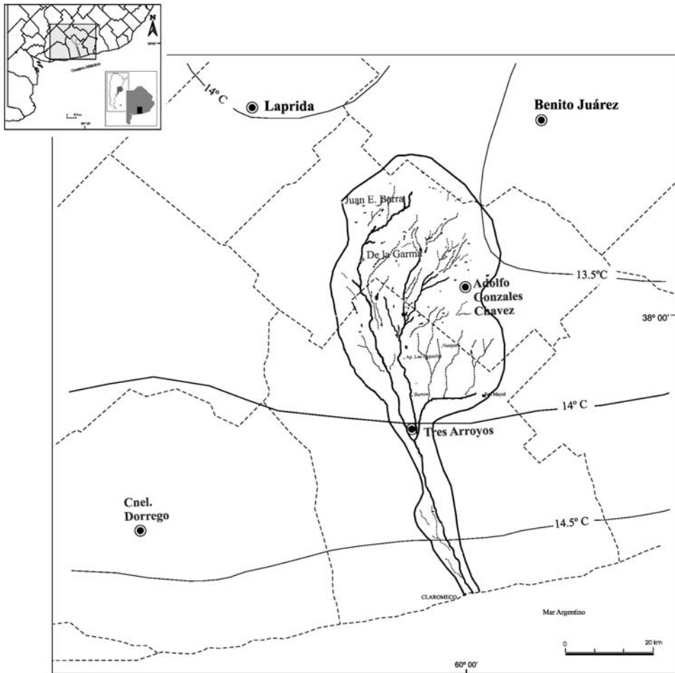
FIGURA 7 Isotermas correspondientes a la cuenca del arroyo Claromecó
