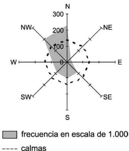
FIGURA 14 Rosa de los vientos de la localidad de Tres Arroyos. Período 1981/1990
