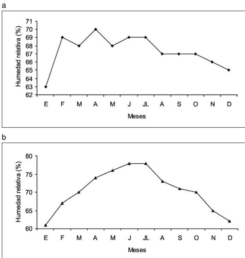
FIGURA 12 Humedad relativa media a. Laprida y b. Tres Arroyos. Período 1981/1990
