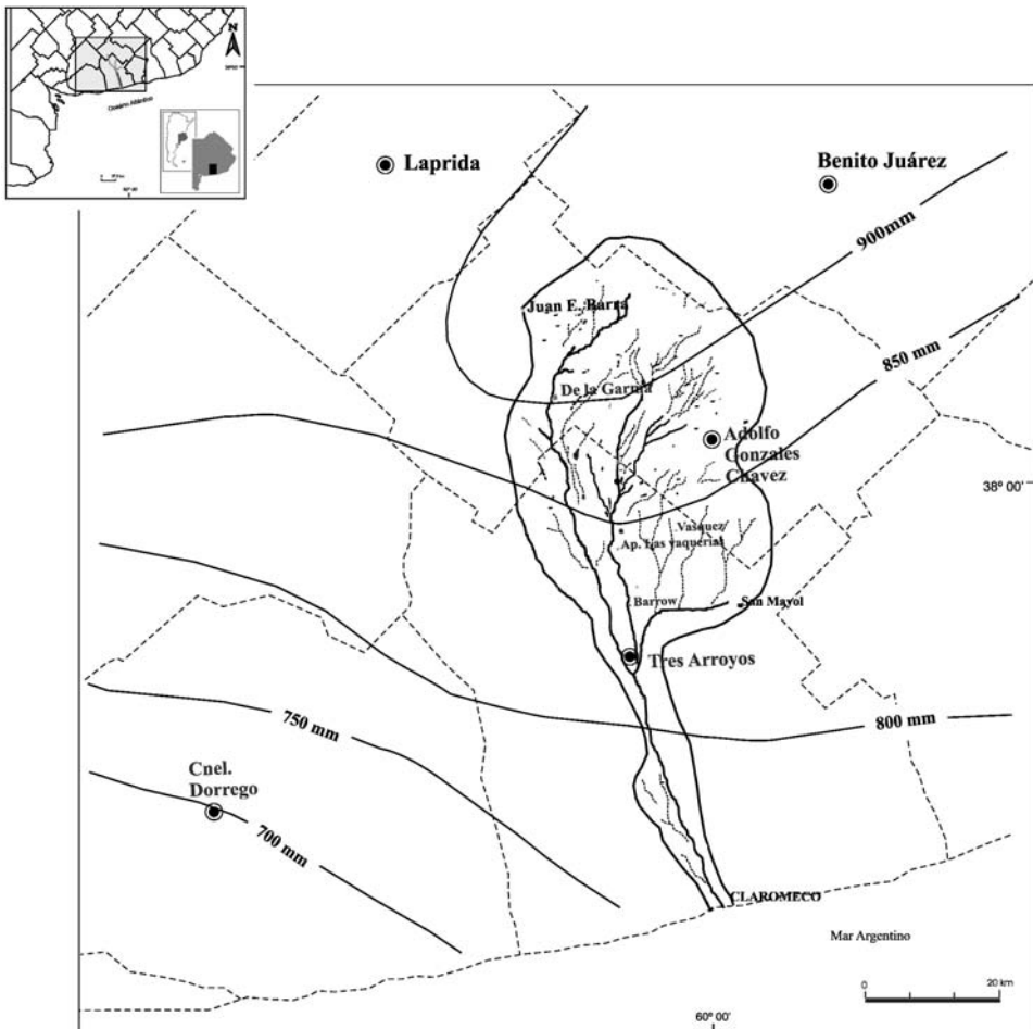
Mapa de isoyetas correspondientes a la cuenca del arroyo Claromecó (1981/1990)
