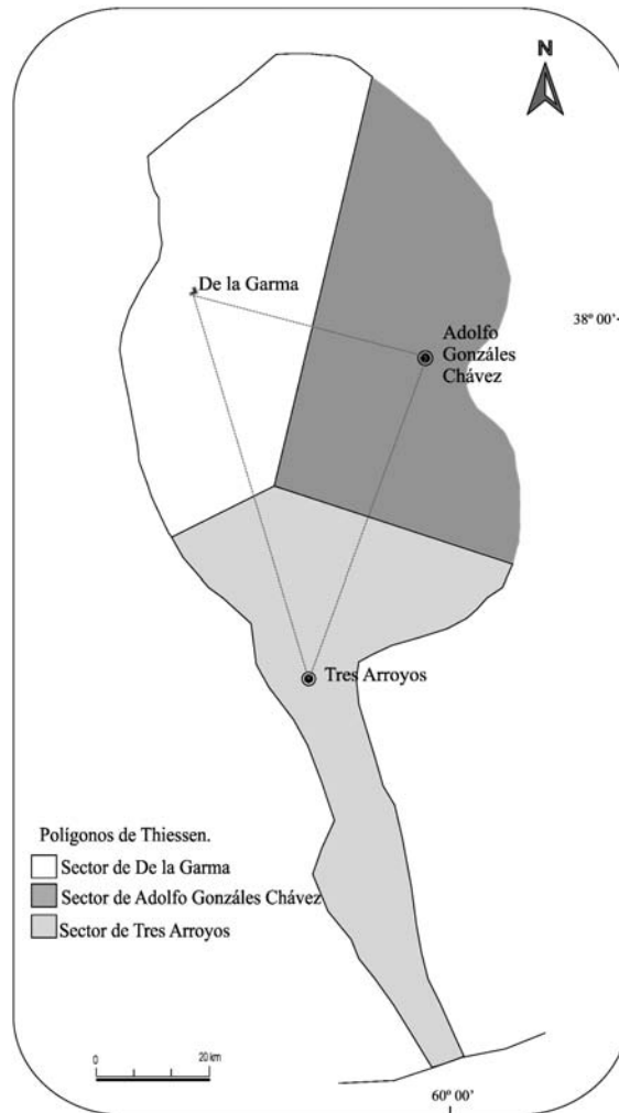
FIGURA 3 Cálculo de la precipitación promedio sobre la cuenca de acuerdo al método de Thiessen
