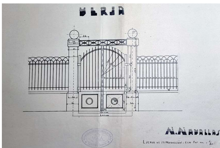
Dibujo de una verja, de Nicolás Navallas, en el Cuaderno de la Escuela de Ampliación de Sangüesa. Año: 1946.
