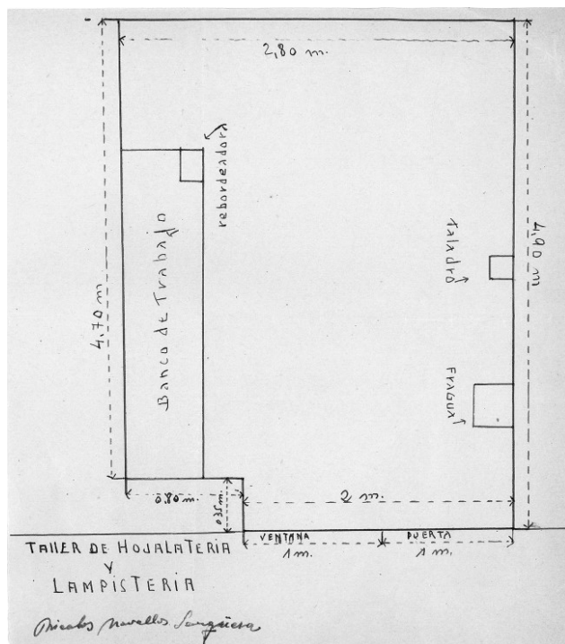
Taller de Hojalatería y Lampistería de Nicolás Navallas en la calle Nueva, nº 32. Croquis realizado por Nicolás Navallas. Año: 1950
