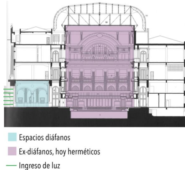
Fig 17. Estación Julio Prestes. Espacios diáfanos e ingreso de luz. Elaboración propia.
