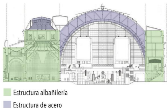
Fig 10. Musée d'Orsay. Esquema de estructuras en corte. Elaboración propia.
