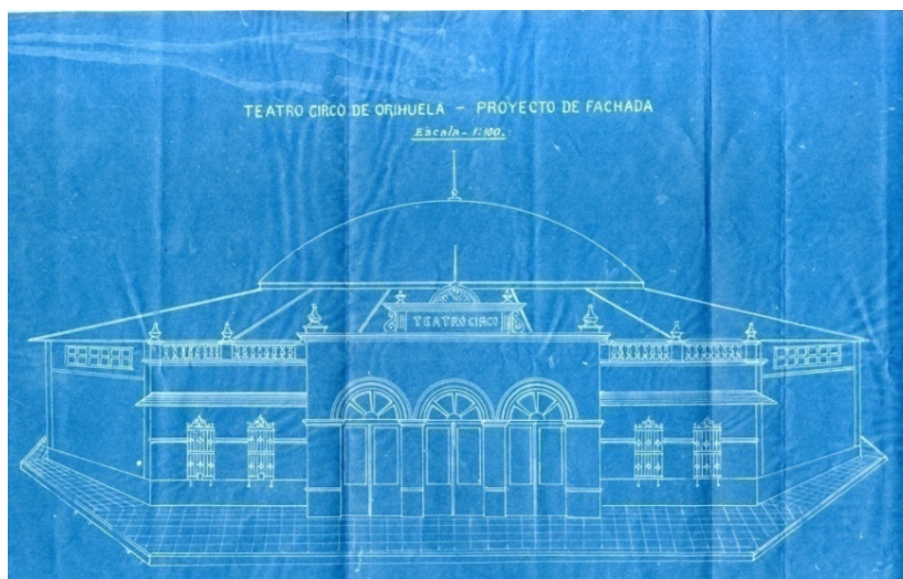
Figura 8. Alzado en perspectiva del Teatro-Circo de Orihuela
