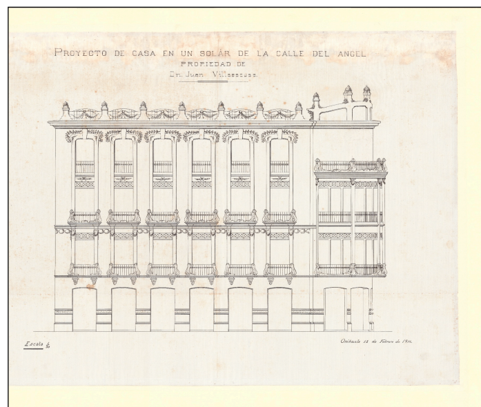
Figura 10. Fachada lateral de la Casa Villaescusa, obra de Joaquín Sánchez Ballesta
