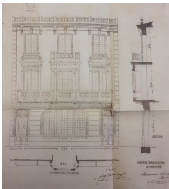
Figura 20. Fachada del edificio de viviendas sito en la Calle San Pascual
