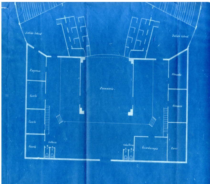
Figura 9b: Plano parcial del escenario del Teatro Circo de Orihuela
