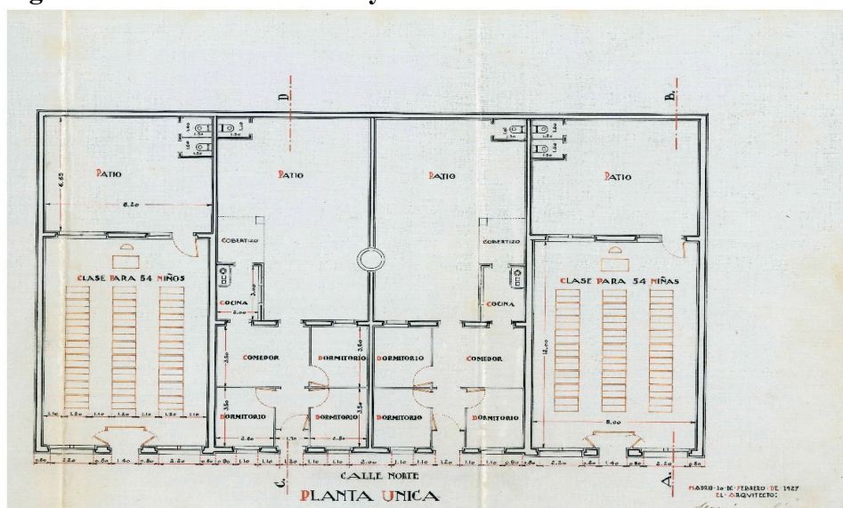
Figura 17. Planta de las aulas y viviendas de las Escuelas de Almoradí
