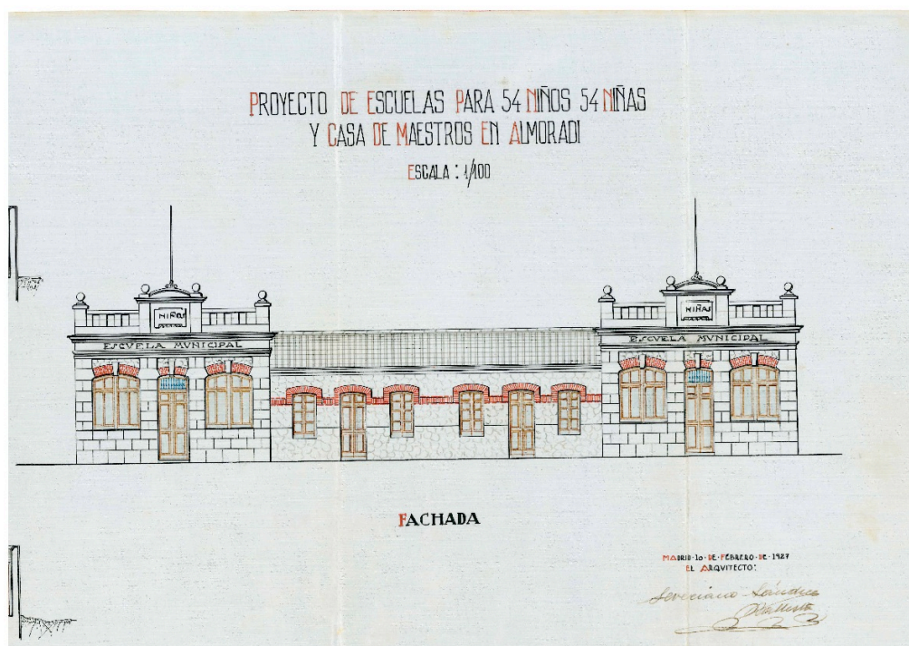
Figura 16. Fachada de las Escuelas de Almoradí
