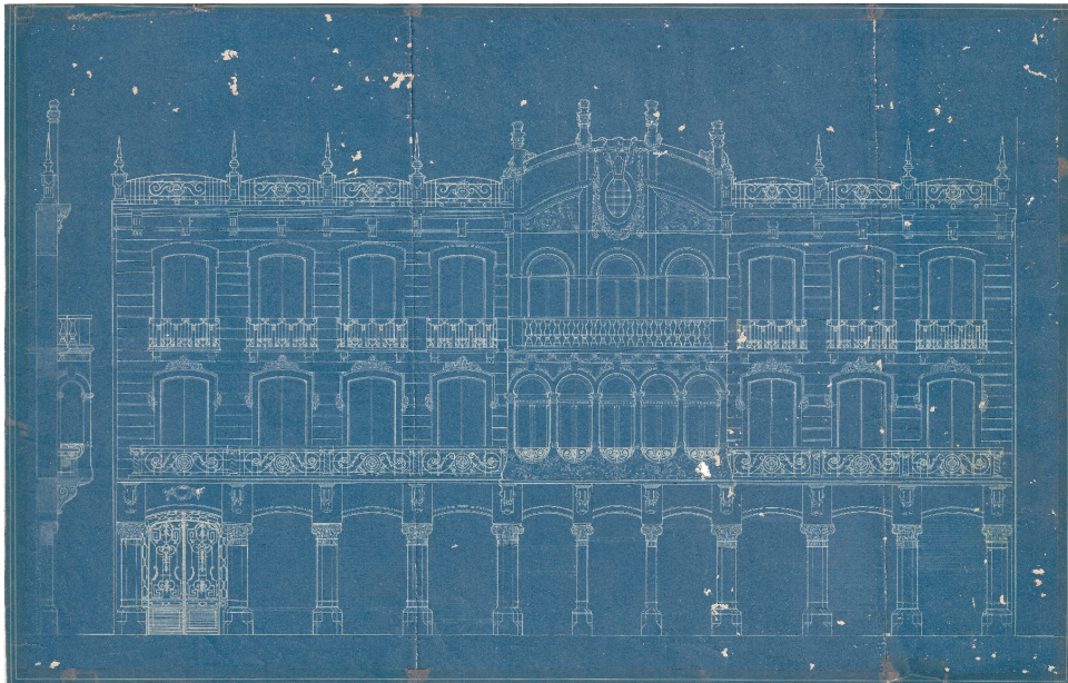
Figura 22. Alzado del edificio modernista de la Casa Martínez-Canales
