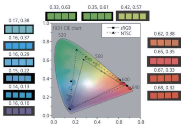
Figura 1. Trazado coordenadas CIE
