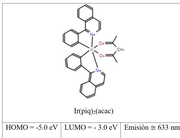
Figura 7. Propiedades del Ir(piq) 2 (acac)
