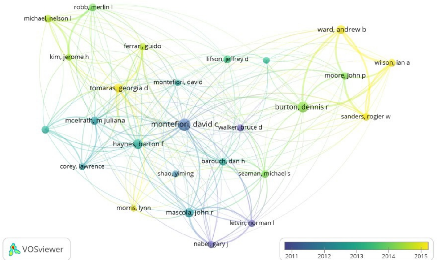
Figura 2. Red de co-ocurrencia de autores(as) con el diseño de Fruchterman-Reingold. Clúster que considera una red de co-ocurrencias entre autores y su progresión en el periodo 2011-2015, graficado según color.
