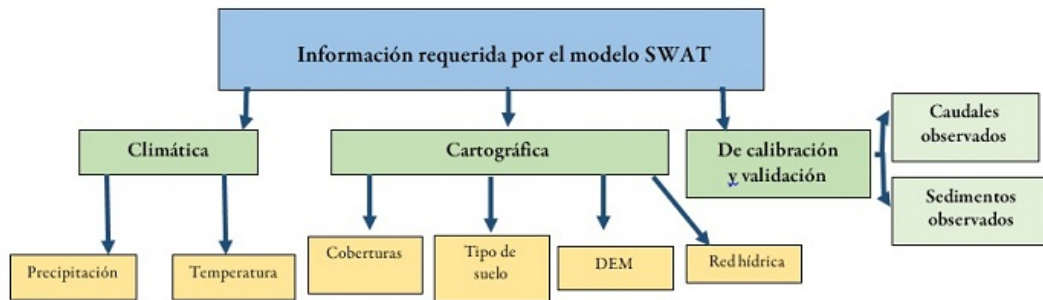
FIGURA 2. Flujoograma de los insumos requeridos por el modelo SWAT Fuente: Ríos (2015, p. 16)
