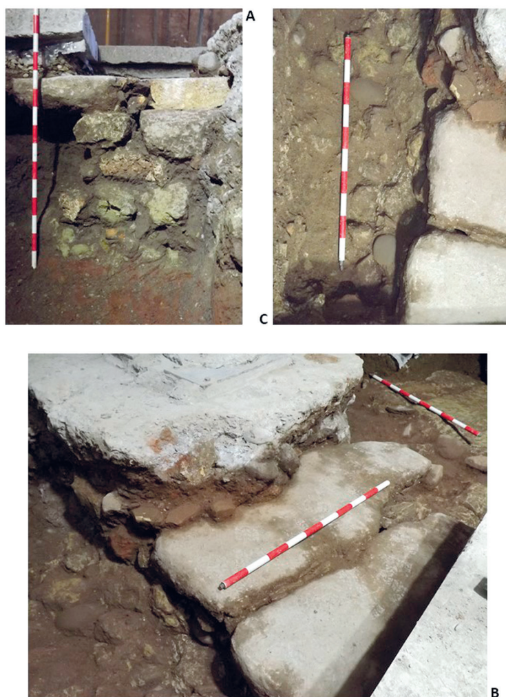
Fig. 4: Cloaca documentada en c/ Duque de Hornachuelos 10. A. Detalle de la fábrica del lateral sur de la cloaca. B. Detalle de la cubierta de la cloaca. C. Detalle del relleno de la zanja de cimentación de la cloaca.
