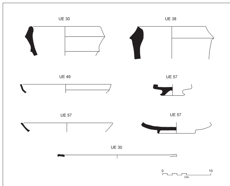
Fig. 7: Material de cronología republicana recuperado en la intervención en c/ Duque de Hornachuelos 10.
