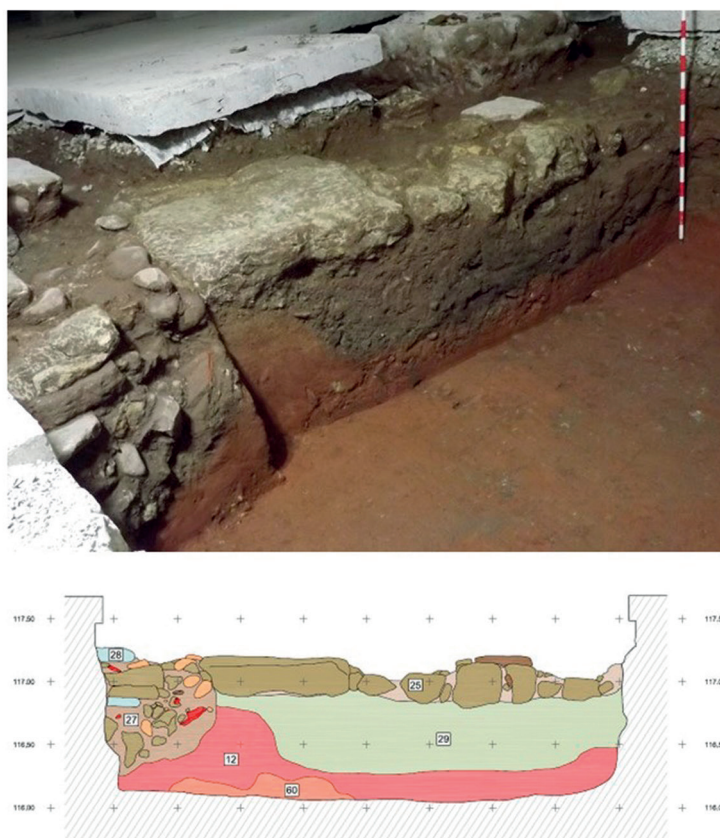
Fig. 5: Fosa rellena de material republicano documentada en c/ Duque de Hornachuelos 10.
