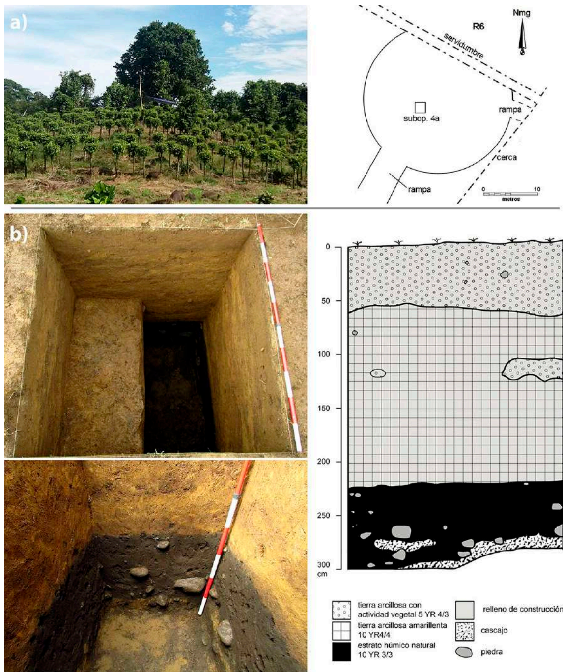
Figura 10: Vista a) desde el suroeste del basamento R5 con plano del contorno, rampas y cala 4a, además de b) perfil de la pared este, fotografía cenital y vista de la parte inferior de la pared norte, complejo Palmeto-Núñez, sitio Anita Grande (fotos y dibujo producidos por J. Brenes, archivo DAH-MNCR).
