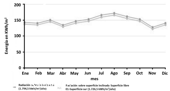
Figura 8. Radiación incidente sobre el arreglo fotovoltaico. Fuente: propia
