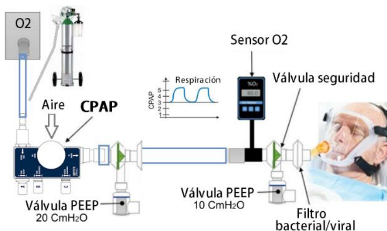
Figura 1: Esquema de funcionamiento del CPAP
