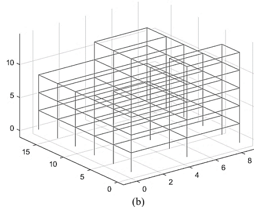
Figura 4. Estructuras irregulares con CEINCI-LAB, a) 2D; b) 3D. Fuente: Los autores.
