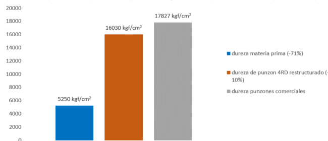
Gráfica 5. Relación de dureza de la materia prima respecto a la dureza de punzón 4RD manufacturado endurecidos y la dureza del promedio de punzones comerciales
