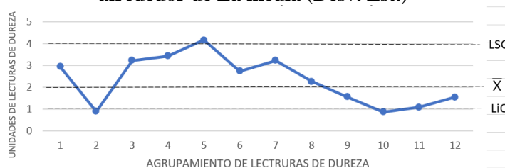
Gráfica 7. Variabilidad de las lecturas de dureza RC Y RB en equipo de medición alrededor de La media (Desv. Est.)
