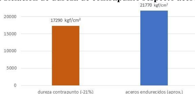
Gráfica 2. Relación de dureza de contrapunto respecto acero endurecidos
