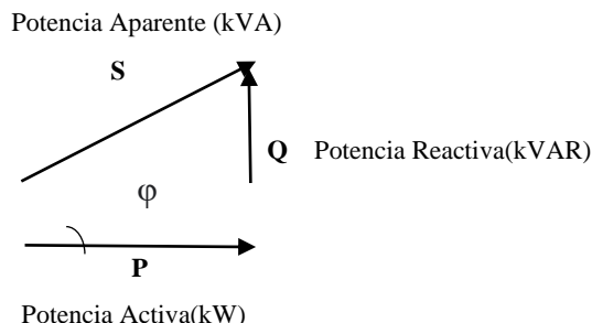
Figura 1. Triángulo de Potencias
