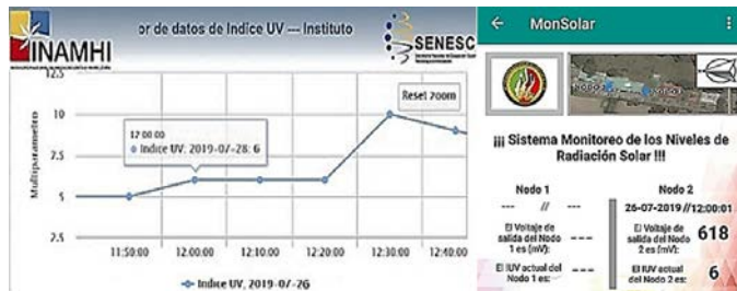
Fig. 18. Gráfica del IUV obtenido, entre INAMHI y el sensor GUYA- S12SD, en función de tres de las horas (11-12-13 horas) con mayor radiación en el día (clima: soleado y semi-templado).
