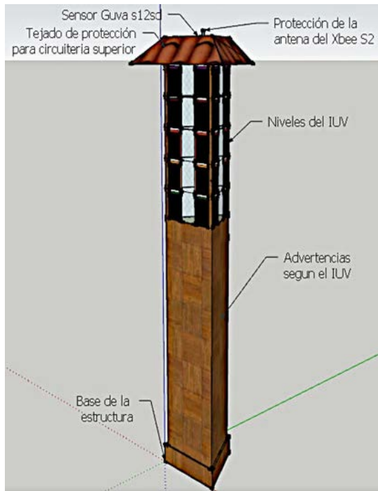
Fig. 7. Diseño de la estructura del solmáforo.
