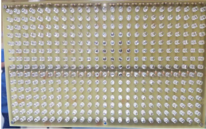
Placa de fototerapia con lámparas LED elaborada por los autores.
