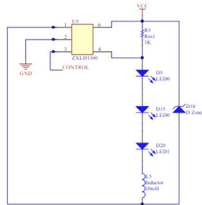
Placa de fototerapia con lámparas LED elaborada por los autores.
