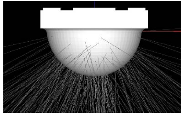
Trazado de los rayos del LED mediante distribución de luz en el espacio de acuerdo al cálculo proporcionado con un ángulo de 140 grados.
