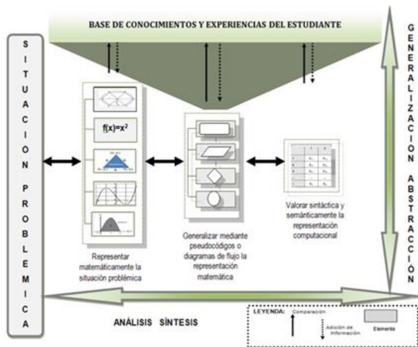
Figura1: Estructura operacional de la habilidad Algoritmizar computacionalmente
