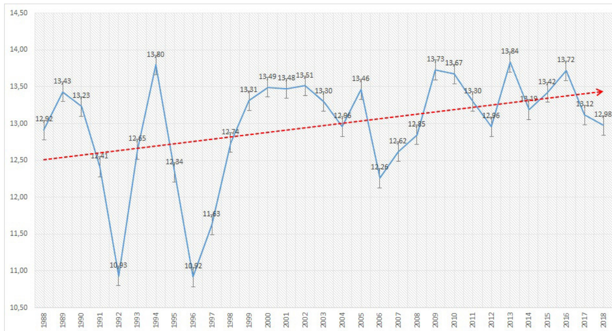
Figura 5. Incremento de temperatura registrada ao longo do período (1988 -2018) sobre a comunidade.
