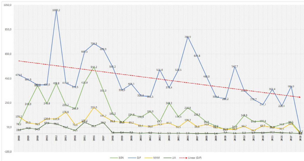
Figura 4. Índice de precipitação de Tentami. Meses: Média trimestral de SON (setembro – outubro e novembro), DJF (dezembro, janeiro e fevereiro), MAM (março, abril e maio) e JJA (junho, julho e agosto).
