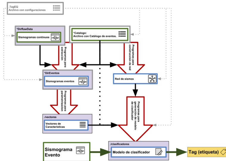
Figura 1. Flujo de datos y arquitectura del sistema
