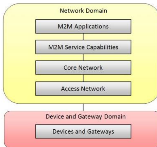
Figura 1. Dominios de la arquitectura funcional M2M de ETSI[14]
