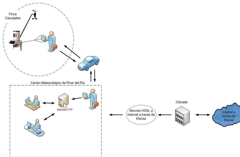
Figura 3. Monitoreo de datos ambientales antes de la solución M2M (elaboración propia)
