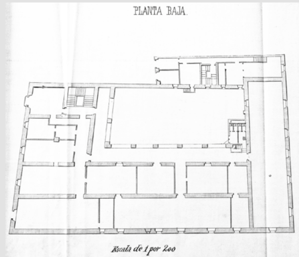
Fig. 9. Planta baja. Celestino Capmany, 1890. Arxiu Diputació de Lleida.
