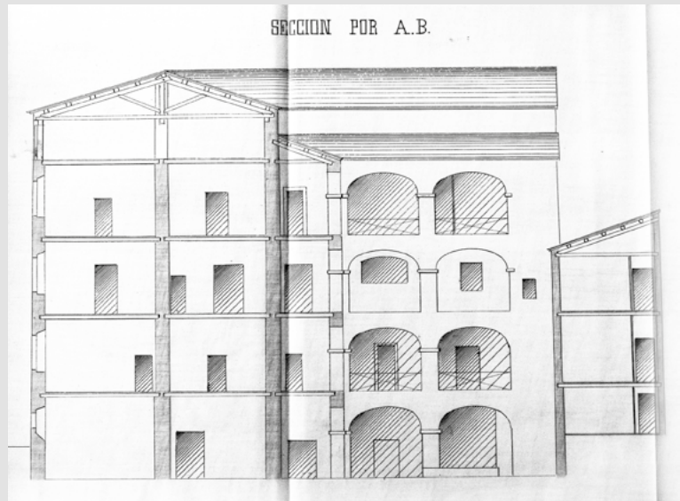
Fig. 7. Sección por A. B, tall perpendicular entre el carrer de l'Audiència i el de la Font d'Aiguadent. Celestino Capmany, 1890. Arxiu Diputació de Lleida.
