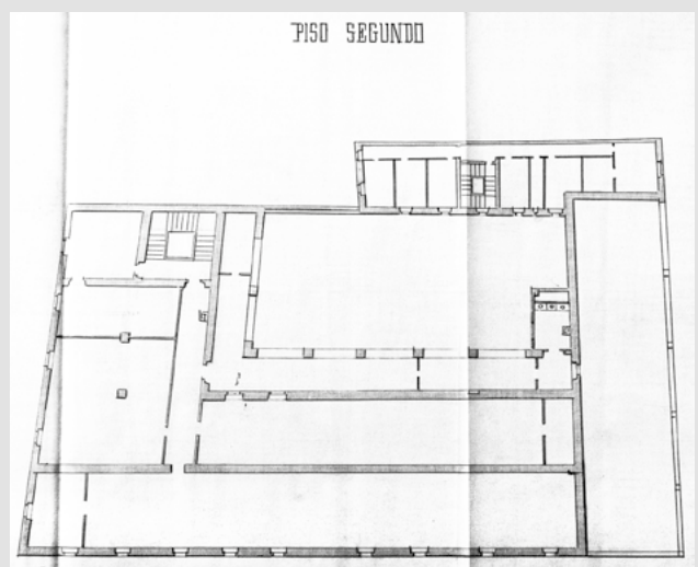
Fig. 11. Piso Segundo. Celestino Capmany, 1890. Arxiu Diputació de Lleida.
