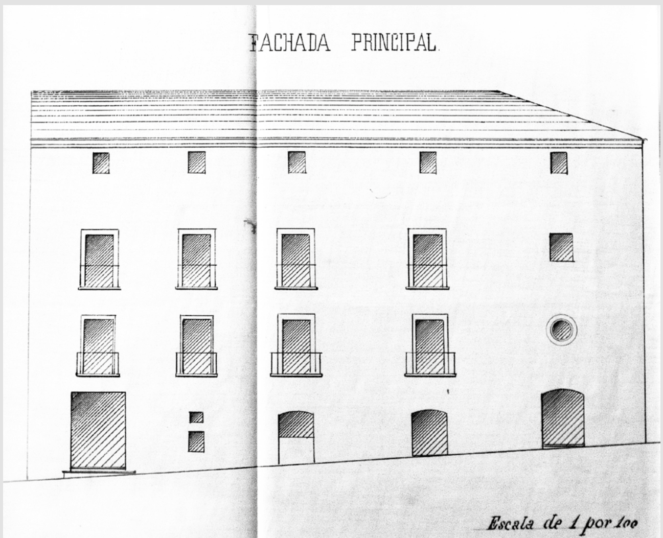
Fig. 13. Fachada lateral. Celestino Capmany, 1890. Arxiu Diputació de Lleida.
