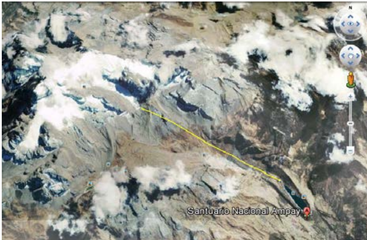
Figura 1. Imagen satelital del nevado Ampay. La línea indica el retroceso del nevado desde el año 1997. Actualmente el área se muestra como zonas rocosas totalmente desnudas
