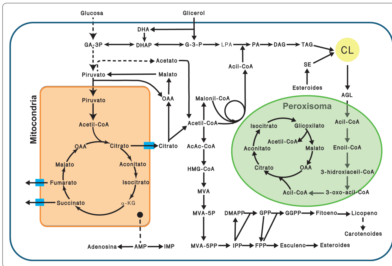
Figura 2. Vías metabólicas de R. toruloides . Glucólisis, ciclo de Krebs en la mitocondria, biosíntesis y degradación de ácidos grasos, triacilglicérol y fosfolípidos, biosíntesis de isoprenoides. Abreviaturas: GA-3P, gliceraldehído-3-fosfato; DHA, dihidroxiacetona; DHAP, dihidroxiacetona fosfato; G3P, glicerol-3-fosfato; LPA, ácido lisofosfatídico; PA, ácido fosfatídico; DAG, diacilglicérol; TAG, triacilglicérol; SE, ésteres de estero; AGL, ácidos grasos libres; CL, cuerpos lipídicos; OAA, oxaloacetato; \alpha -KG, \alpha -cetoglutarato; AcAcCoA, aceto-acetil-CoA; HMG-CoA, hidroximetilglutaril-CoA; MVA, mevalonato; MVA-5P, mevalonato-5-fosfato; MVA-5PP, mevalonato-5-difosfato; IPP, isopentenil difosfato; DMAPP, dimetilalil pirofosfato; GPP, geranil pirofosfato; FPP, farnesil pirofosfato; GGPP, geranilgeranil pirofosfato; AMP, adenosín monofosfato; IMP, inosina monofosfato. Modificada de (Wen et al. , 2020).
