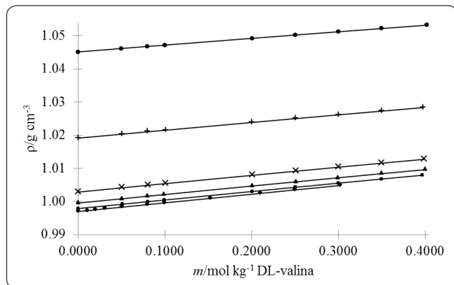
Figura 1. Densidades de la DL-valina en mezclas acuosas de NaNO 3 (□ 0.0000, × 0.0106, ▲ 0.0413, ◆ 0.1009, + 0.4013, • 0.9014) mol kg -1 a temperatura de 298.15 K.
