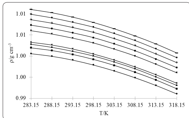
Figura 2. Densidades de la DL-valina en mezcla acuosa de NaNO 3 0.0106 mol kg -1 a diferentes temperaturas. (Todos los sistemas acuosos de NaNO 3 estudiados presentan la misma tendencia en sus datos).
