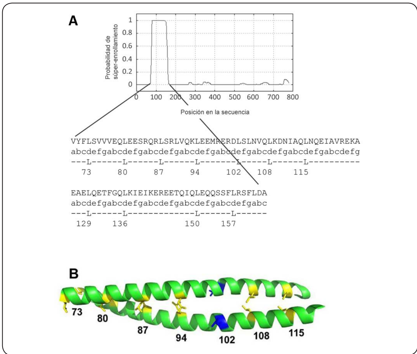
Figura 2. A. Predicción de los motivos súper-enrollados encontrados en la secuencia de ArcB obtenida por la herramienta COILS/PCOILS 38 . Abajo se presenta la secuencia del motivo de ArcB, con repeticiones hepta-peptídicas de leucinas. B. Modelo de ArcB de la secuencia 73 a 121, generado sobre la estructura cristalina de un modelo dimérico súper-enrollado (Código PDB 3he5). Los residuos de leucina en las posiciones 73, 80, 87, 94, 108 y 115 están indicados en color amarillo y la posición de la leucina 102 en color azul (Reproducido de Núñez et al, 2012) 15 .
