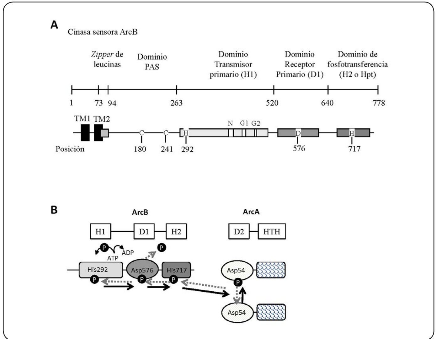
Figura 1. A. Representación esquemática de la cinasa sensora ArcB. B. Representación esquemática de las reacciones de fosforilación de ArcB. Flechas sólidas indican la vía de transferencia del grupo fosforilo que resulta en ArcA-P; flechas punteadas representan el fosforelevo reverso que resulta en la defosforilación de ArcA-P.
