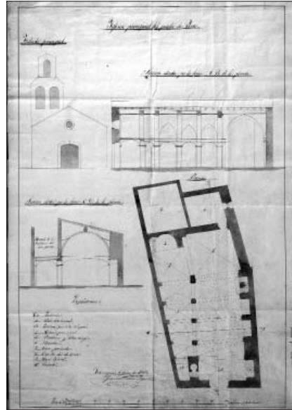
Plànol de l'església parroquial de Pira (AHAT)
