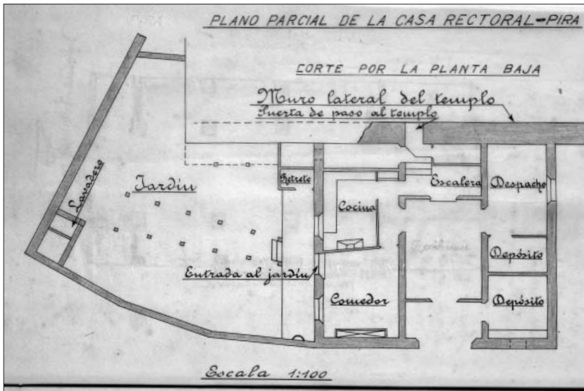
Plànol de la rectoria de Pira (AHAT)
