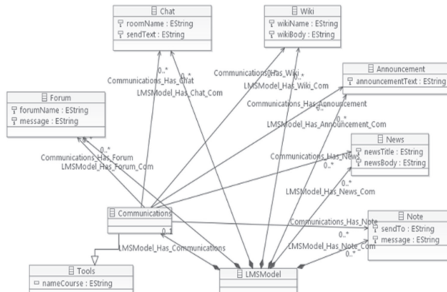
Figura 3 Metamodelo LMS de módulos de comulación.
