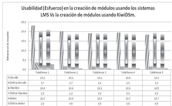
Figura 12 Esfuerzo (usabilidad) en la creación de módulos usando los sistemas LMS Vs la creación de los mismos módulos con la herramienta DSM.
