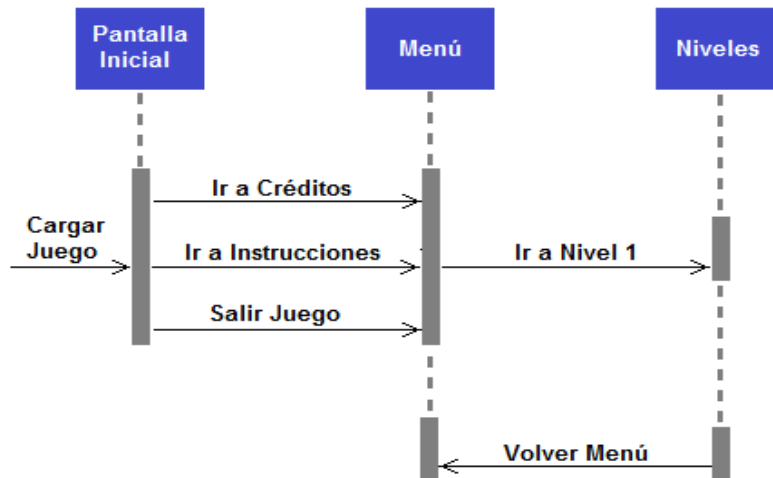
Fig. 3. Diagrama de secuencia iniciar videojuego. Fuente: elaboración propia.
