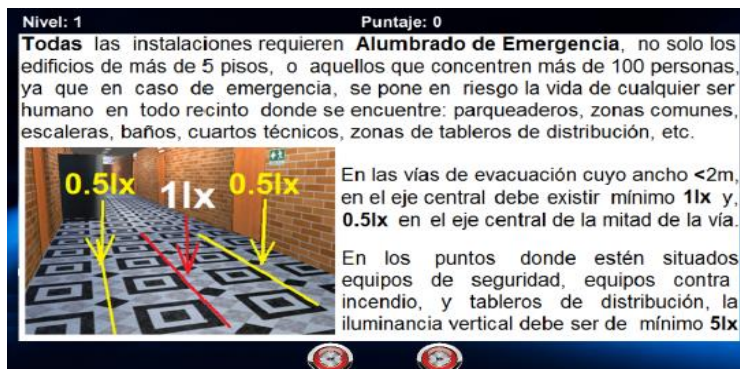
Fig. 23. Explicación de los niveles de iluminación que el RETILAP exige, nivel 5. Fuente: elaboración propia.
