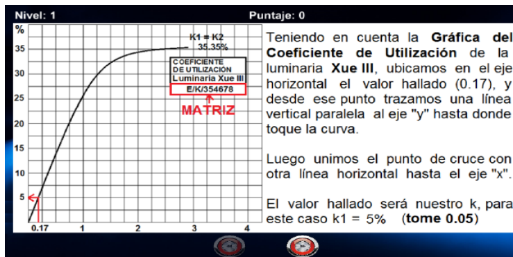
Fig. 17. Explicación del cómo utilizar la gráfica del Coeficiente de Utilización de las luminarias, en el nivel 3. Fuente: elaboración propia.
