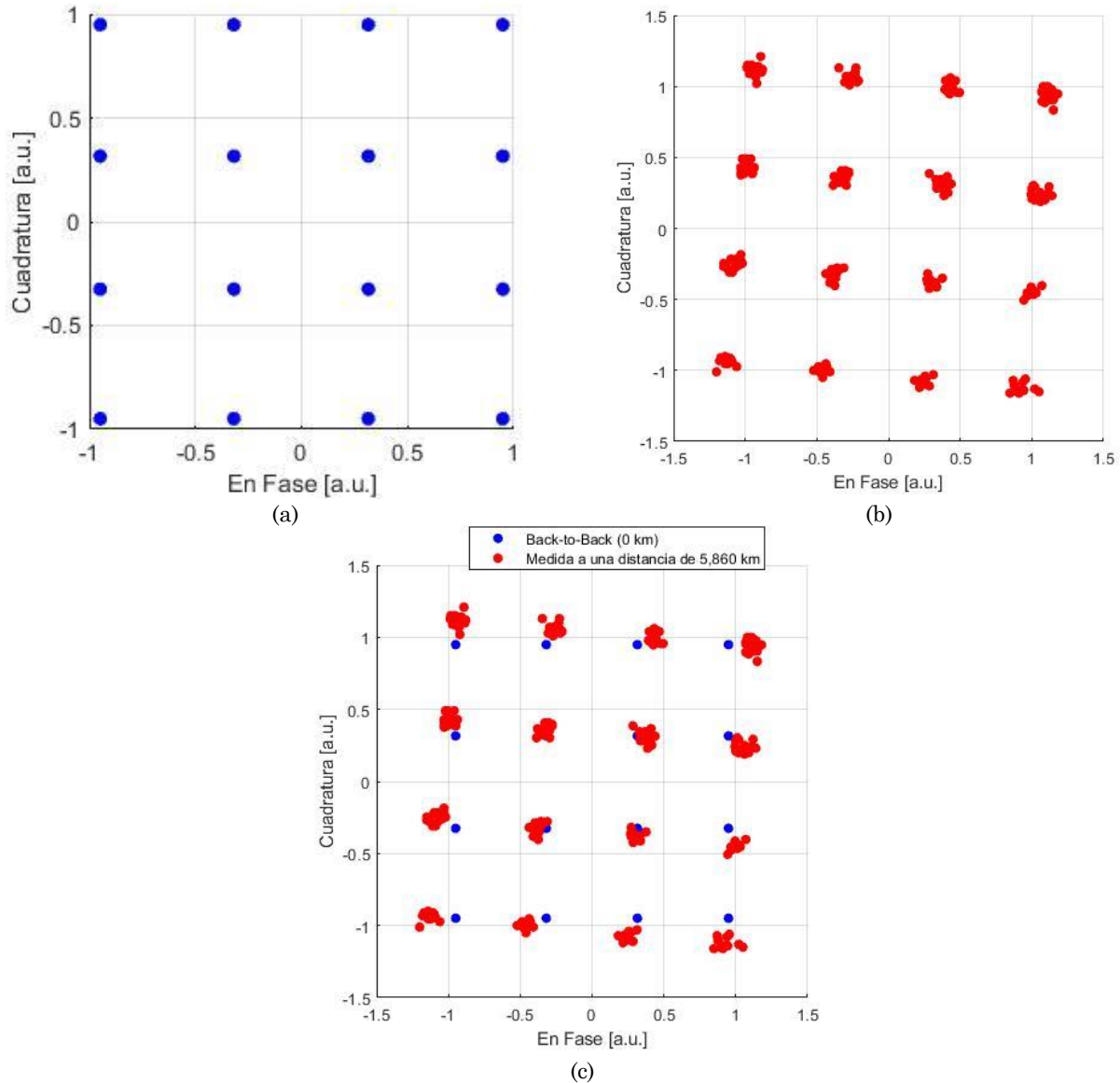
Fig. 16. Diagrama de constelación (en fase y cuadratura) de la señal radio. (a) Back-to-back (0 km). (b) Medida a una distancia de 5,860 km. c) Superpuesto: ideal vs recibido. Fuente: elaboración propia.
