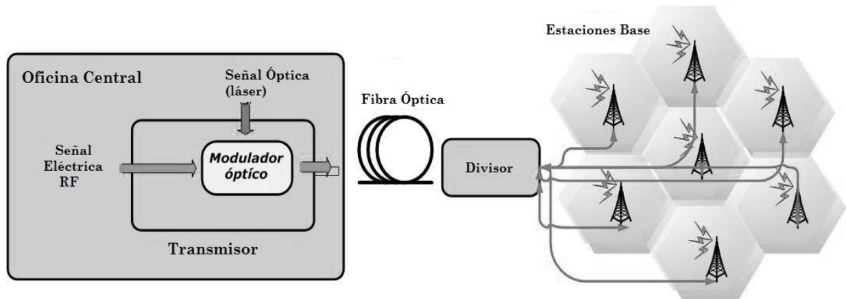
Fig. 2. Sistema RoF. Fuente: [3].
