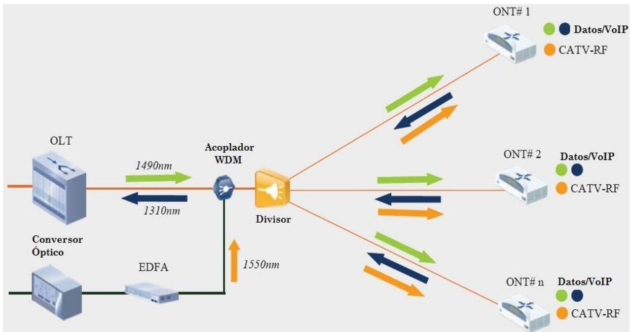
Fig. 1. Esquema de red FTTH-GPON. Fuente: [15].
