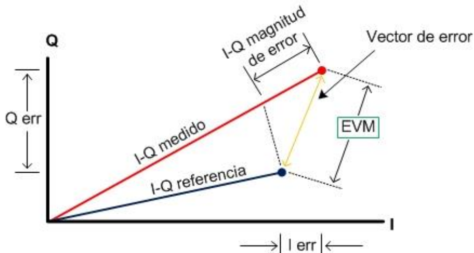
Fig. 13. Representación gráfica de la EVM. Fuente: [27].
