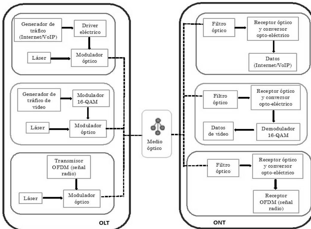
Fig. 11. Modelo conceptual de la red FTTH-GPON Quad Play (con el módulo RoF integrado)
