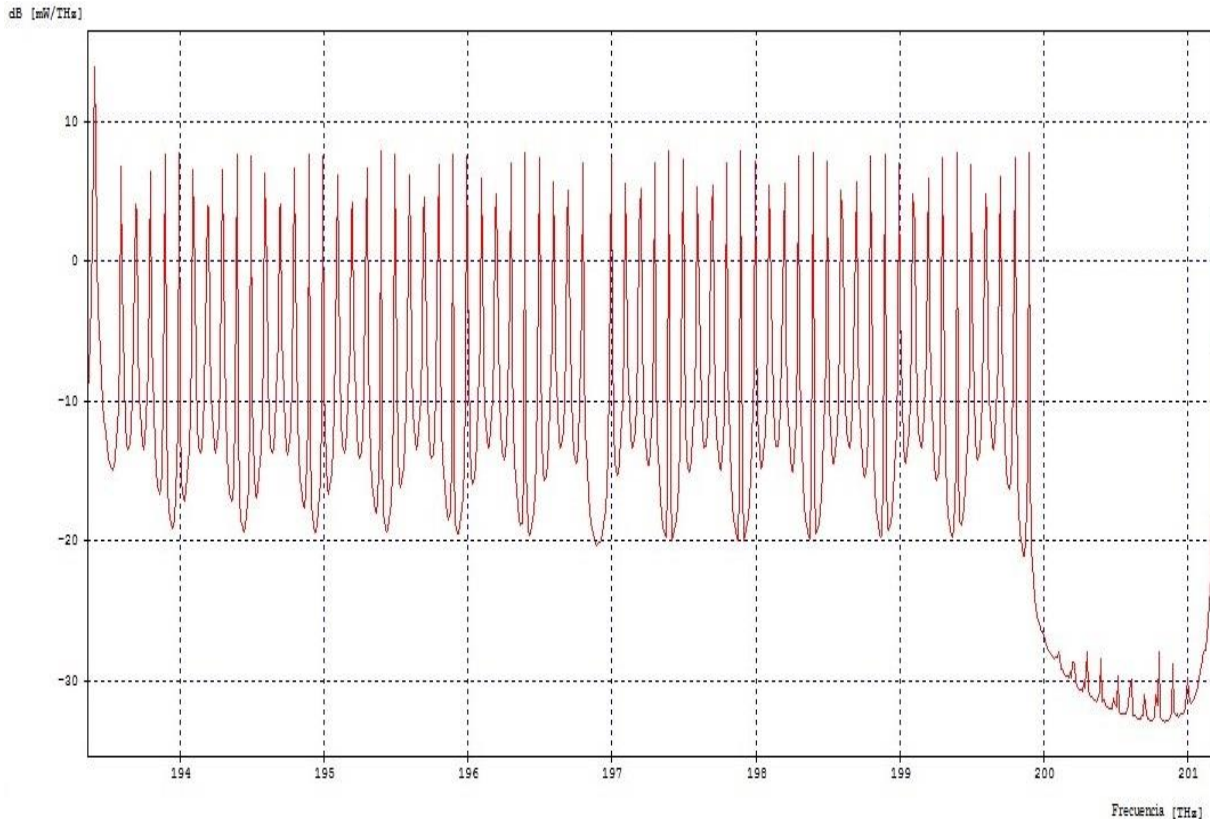
Fig. 25. Espectro de frecuencias para de la red FTTH-GPON Quad Play para 64 ONT Fuente: elaboración propia.
