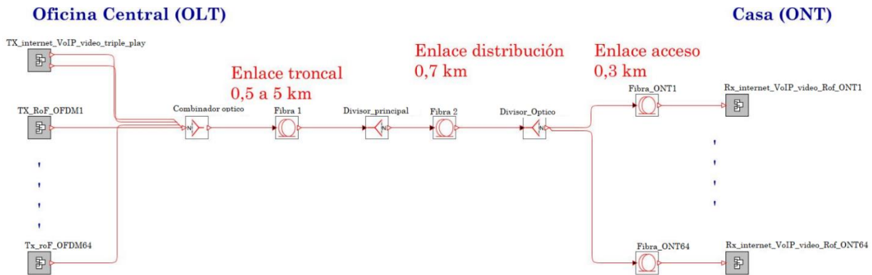
Fig. 24. Modelo general del sistema FTTH-GPON Quad Play para 64 ONT Fuente: elaboración propia.
