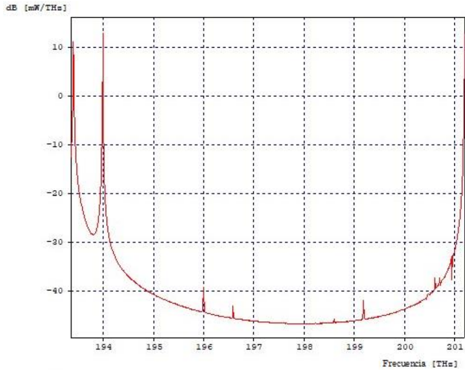
Fig. 20. Señales Quad Play (datos/voz, video y radio) en el canal óptico Fuente: elaboración propia.
