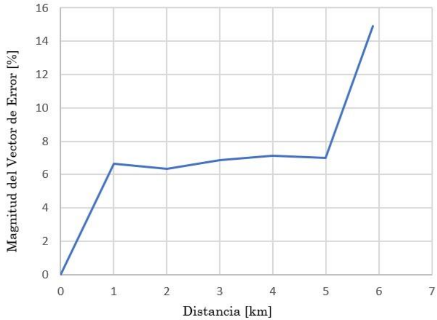
Fig. 22. Variación de la EVM con la distancia para la señal radio medida en el receptor Fuente: elaboración propia.
