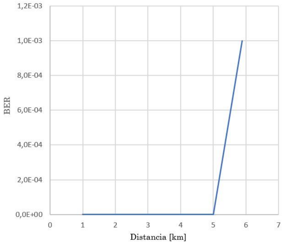
Fig. 23. Variación de la BER con la distancia para la señal radio medida en el receptor Fuente: elaboración propia.
