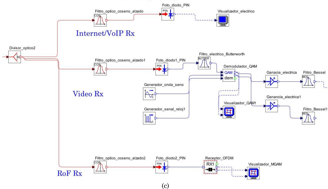
Fig. 12. Modelo físico de la red FTTH-GPON Quad Play (con el módulo RoF integrado) para una sola ONT (a) Transmisor (OLT). (b) Medio óptico. (c) Receptor (ONT). Fuente: elaboración propia.
