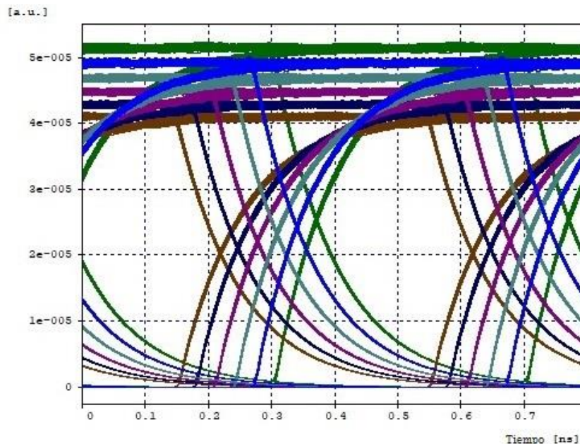
Fig. 17. Variación del diagrama del ojo con la distancia para la señal de datos/voz medida en el receptor Fuente: elaboración propia.
