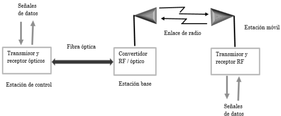
Fig. 4. Configuración de un sistema de comunicaciones RoF. Fuente: [16].
