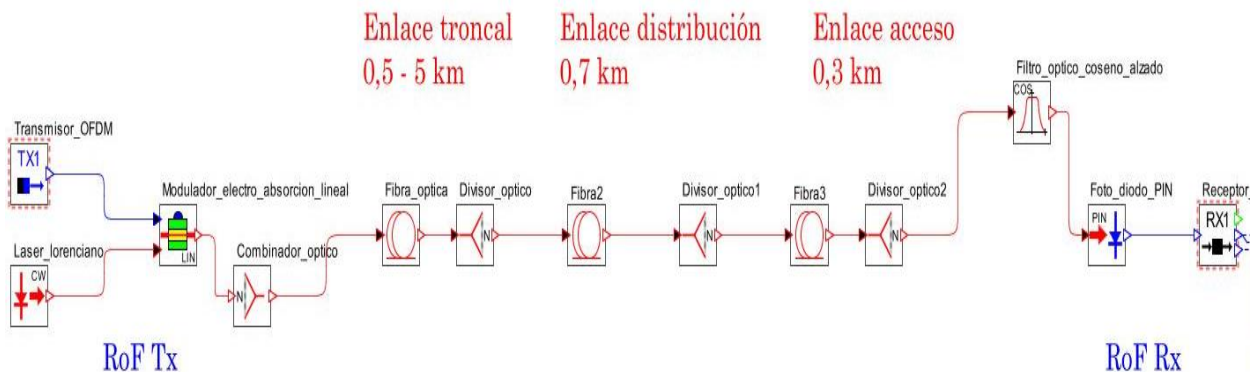
Fig. 9. Modelo físico del módulo RoF para una OLT y ONT Fuente: elaboración propia.
