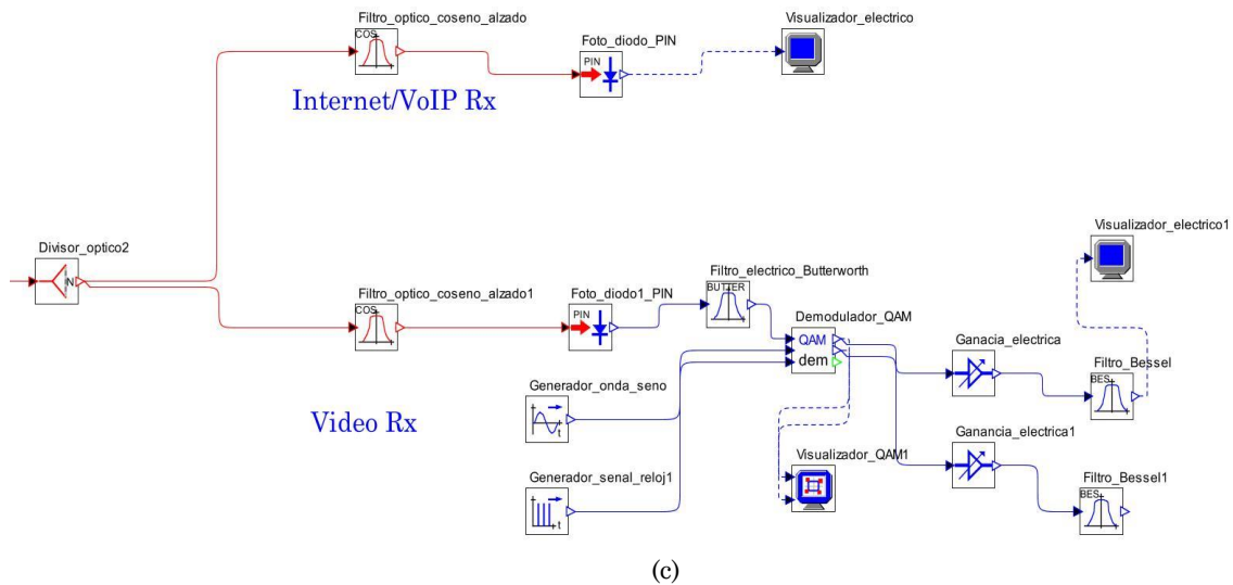
Fig. 7. Modelo físico de la red FTTH-GPON Triple Play (sin el módulo RoF) para una ONT. (a) Transmisor (OLT). (b) Medio óptico. (c) Receptor (ONT). Fuente: elaboración propia.
