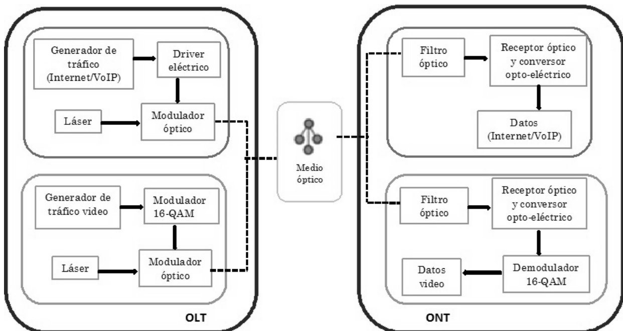
Fig. 6. Modelo conceptual de la red FTTH-GPON Triple Play (sin el módulo RoF). Fuente: [24].
