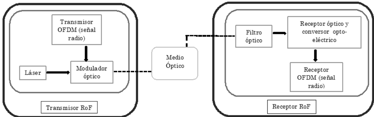
Fig. 8. Modelo conceptual del módulo RoF. Fuente: [16].
