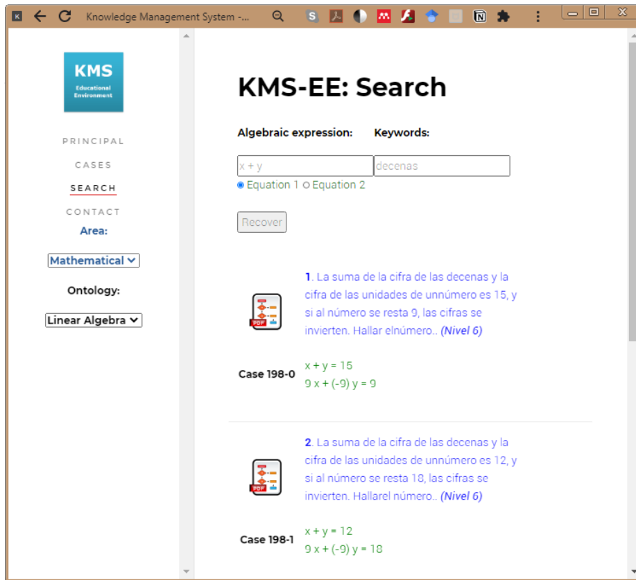
Figura 4. Implementación de SGC adaptado al entorno educativo.
