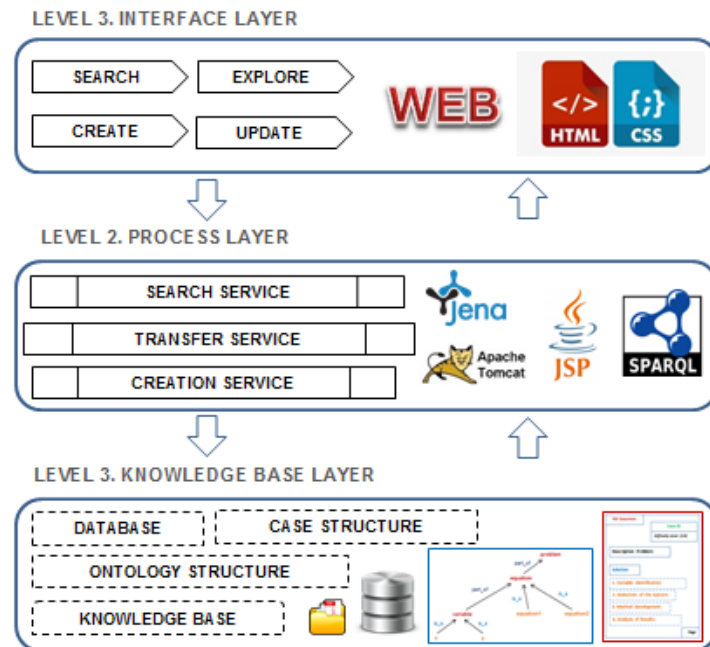
Figura 1. Arquitectura de un SGC basado en ontologías y basado en casos.
