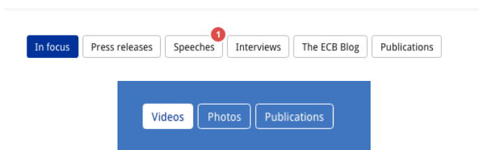
Figura 10: Botones
