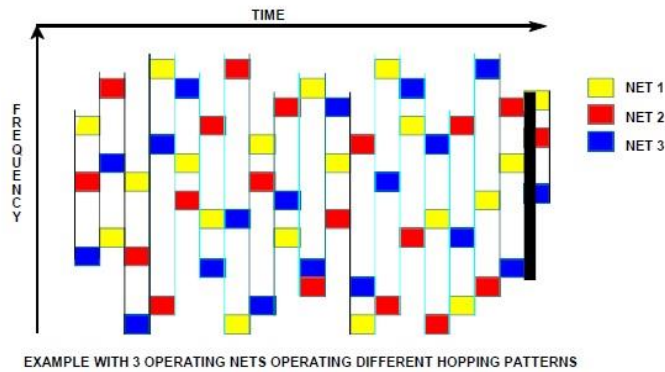
Figura 4. Multiplexación por secuencia de saltos.
