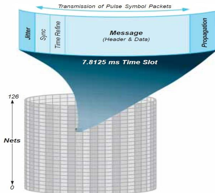
Figura 6. Time slot.
