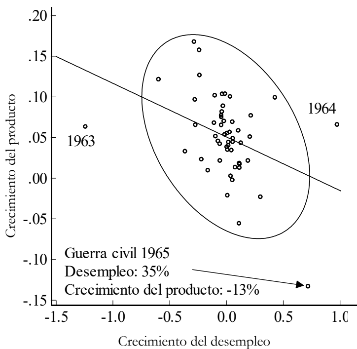
Figura N.º 3 Crecimiento del producto real y del desempleo Diferencia de logaritmos, con elipse y línea de regresión, 1961-2013
