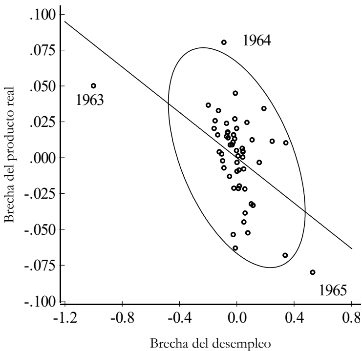
Figura N.º 4 Brechas del producto real y del desempleo Diferencia de logaritmos, con elipse y línea de regresión, 1961-2013
