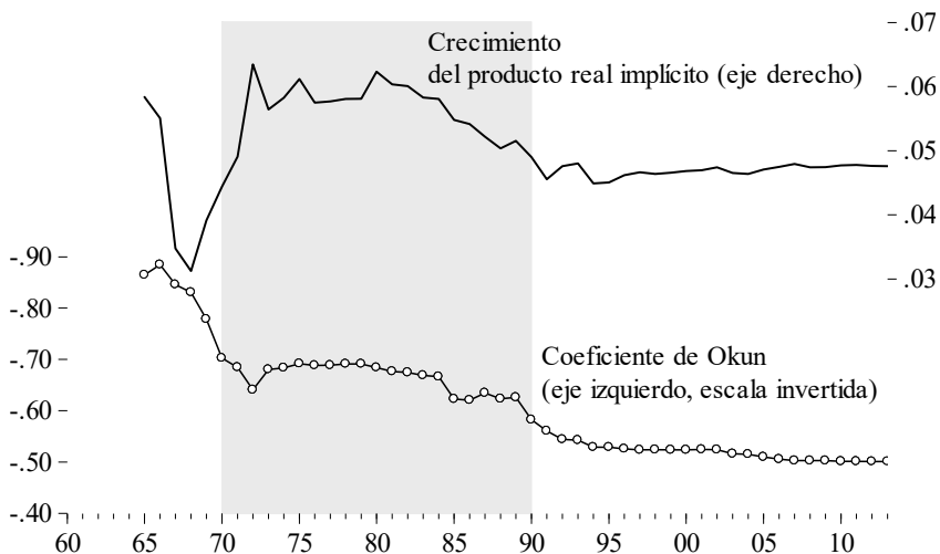
Figura N.º 7 Coefficiente de Okun y valores del producto real consistentes con desempleo estable Estimación recursiva de la ecuación 10, 1965-2013
