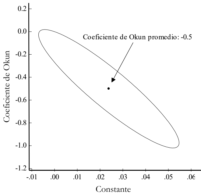
Figura N.º 6 Elipse de confianza de 1% para el coeficiente de Okun, ecuación 10
