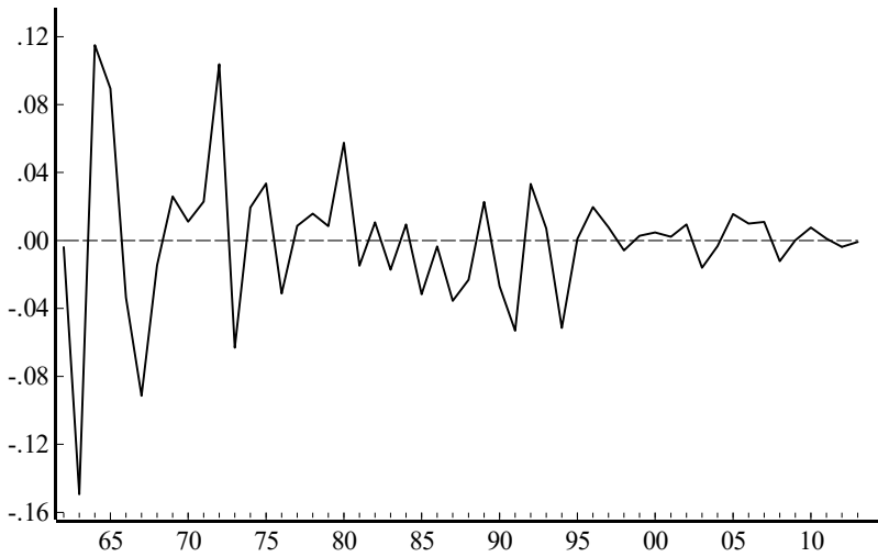
Figura N.º 5 Residuos de la ecuación de Okun número 10, 1962-2013
