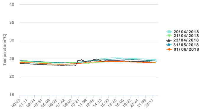
Fig. 12 temperature in geomembrane.
