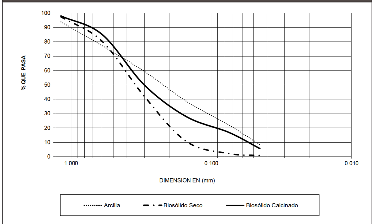
Figura 1. Curva Granulométrica de arcillas y biosólidos (seco y calcinado)
