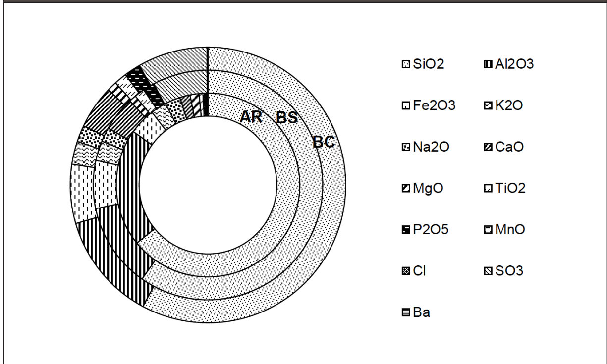
Figura 2. Análisis de la composición química de arcillas y biosólidos A. comparación química de materias primas (Arcilla AR, Biosólidos seco BS y Biosólido calcinado BC)
