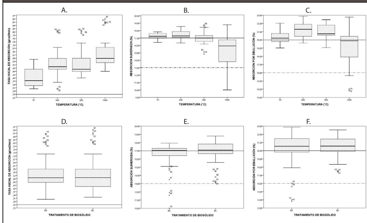
Figura 3. Absorciones de ladrillos cerámicos con biosólidos de aguas residuales en función de las temperaturas (800°C, 900°C, 1000°C y horno), A) Absorción capilar ABSC, B) Absorción sumergida (ABSS) y C) Absorción por ebullición ABSE, en función del tratamiento del biosólido D) ABSC, E) ABSS, F) ABSE
