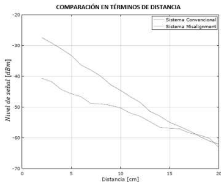
Figura 6. Comparación en distancia de sistemas SCMR Convencional y Misalignment
