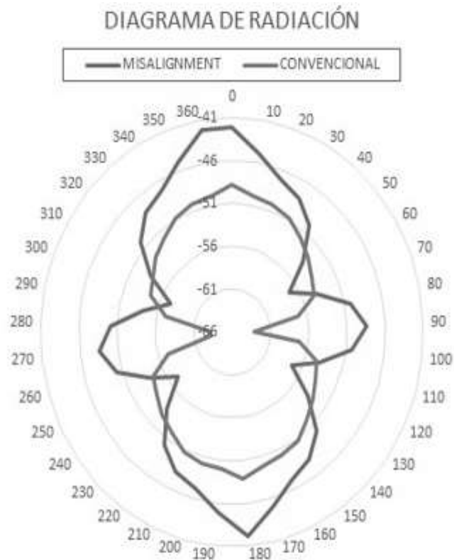
Figura 7. Comparación en alineación de sistemas SCMR Convencional y Misalignment.
