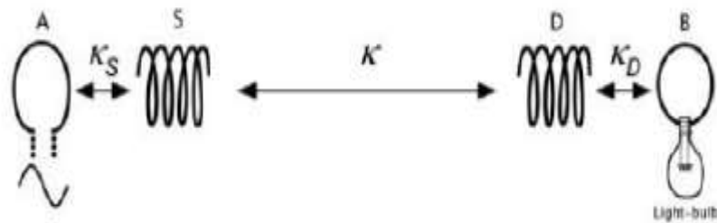
Figura 1. Modelo WTP planteado por el MIT [1].
