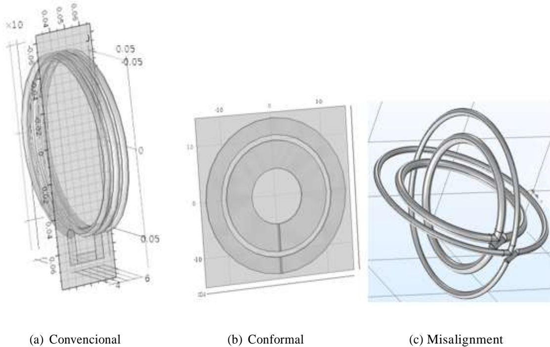
Figura 4. Modelos implementados en el software de simulación
