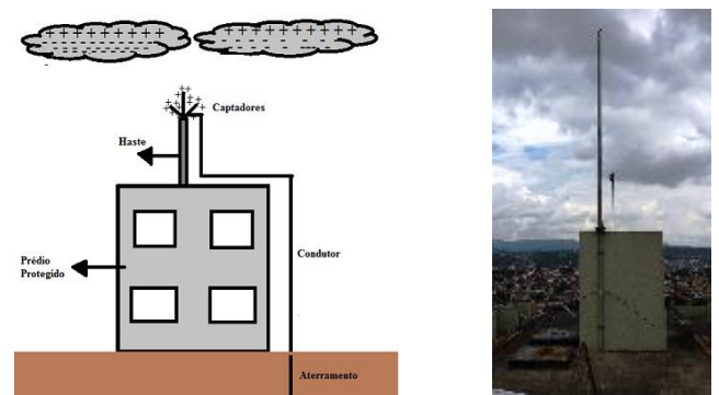
FIGURA 6. Em (a), à esquerda, apresentamos o esquema de um para-raios [26] e, em (b), à direita, apresentamos a imagem da haste vertical do para-raios. Imagem do arquivo pessoal dos autores.
