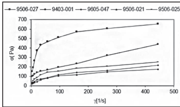
Figura 2. Comportamiento de los almidones de ñame ( D. alata ) a esfuerzos de corte.
