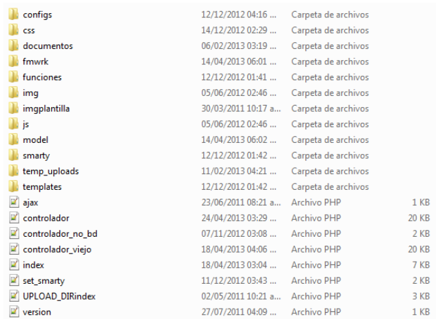
Fig. 13. Estructura de directorios en una aplicación web desarrollada con el Framework de PISIS. Fuente: PISIS
