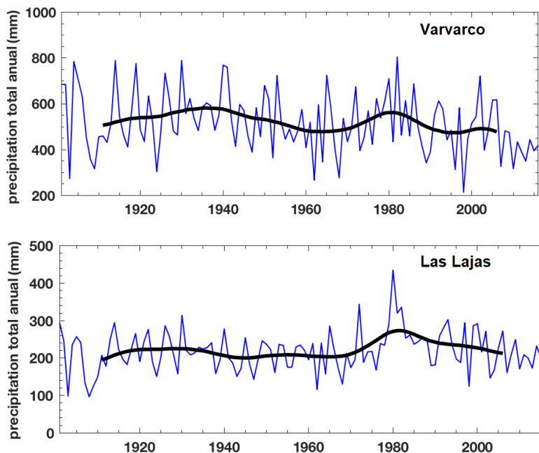
Figura 3. Precipitación anual total (mm) para las estaciones Varvarco y Las Lajas a partir de la base de datos CRUTEM4-2018-06, la línea negra presenta la línea suavizada de 20 años. (Harris, Jones, Osborn, & Lister, 2014).
