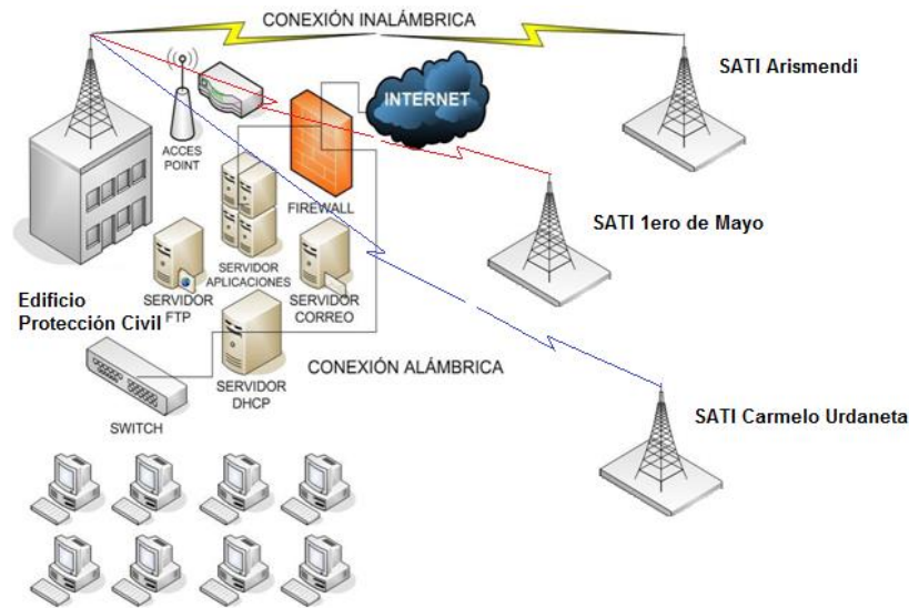
Figura 3: Dispositivos que interactúan entre los enlaces Fuente: Propia (2017)
