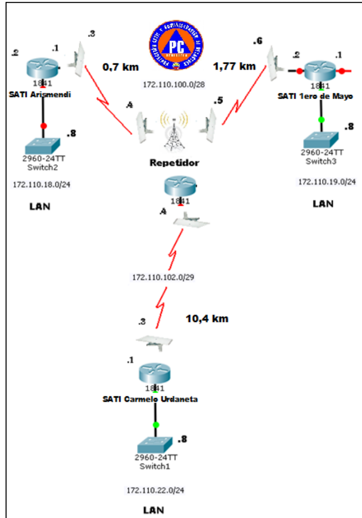
Figura 1: Topología estrella recomendada Fuente: Propia (2017)
