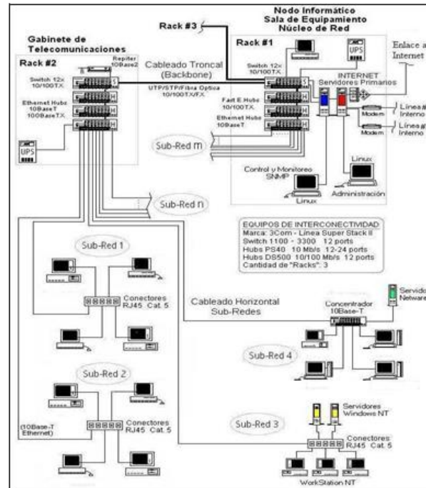
Figura 5: Estructura de gabinetes (Racks) Fuente: Propia (2017)
