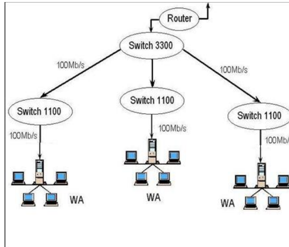
Figura 4: Diagrama jerárquico Fuente: Propia (2017)
